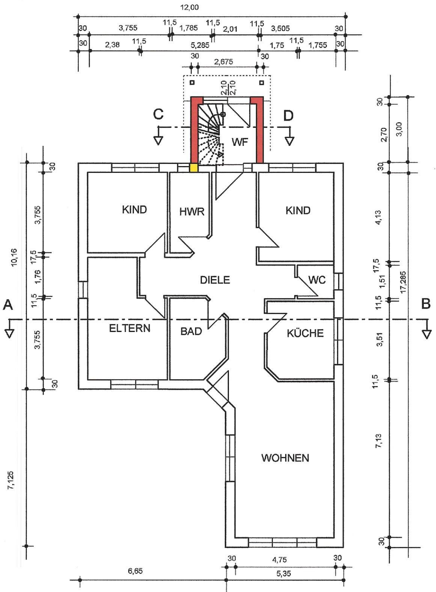
ERDGESCHOSS
