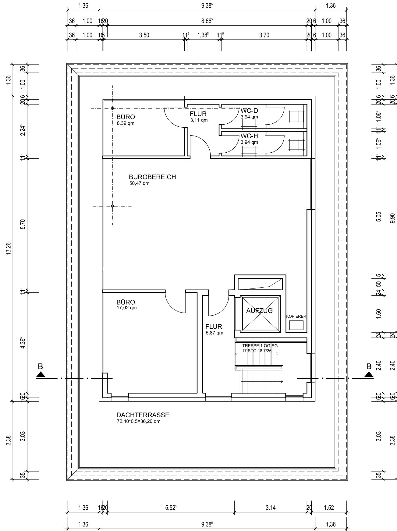
GRUNDRISS STAFFELGESCHOSS
