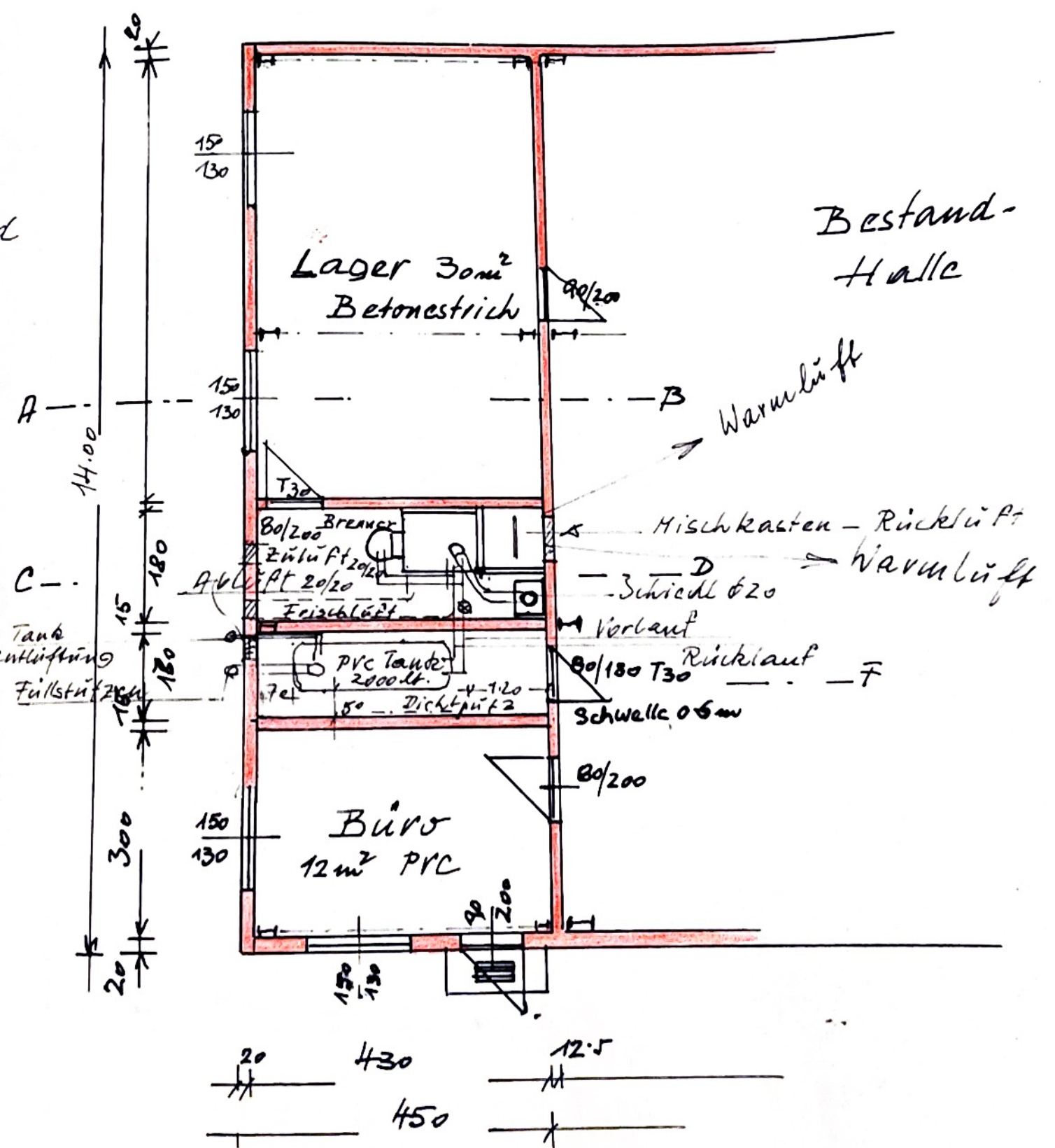
Grundriss M. 1: 100
