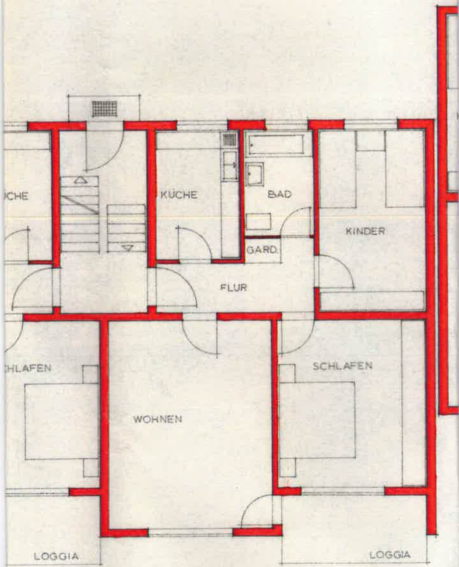
BLOCK 4 3-geschossig
