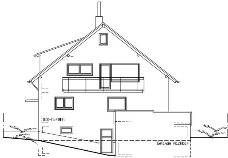
Ansicht Nordwesten
