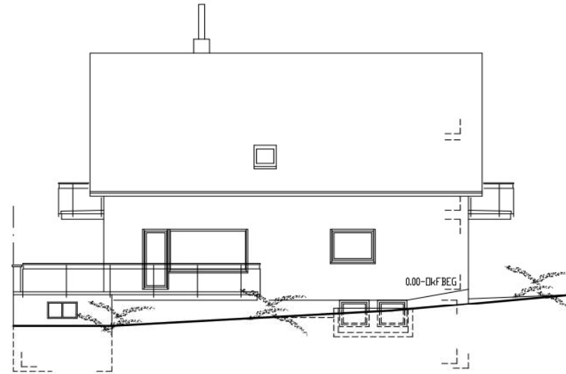
Ansicht Südwesten
