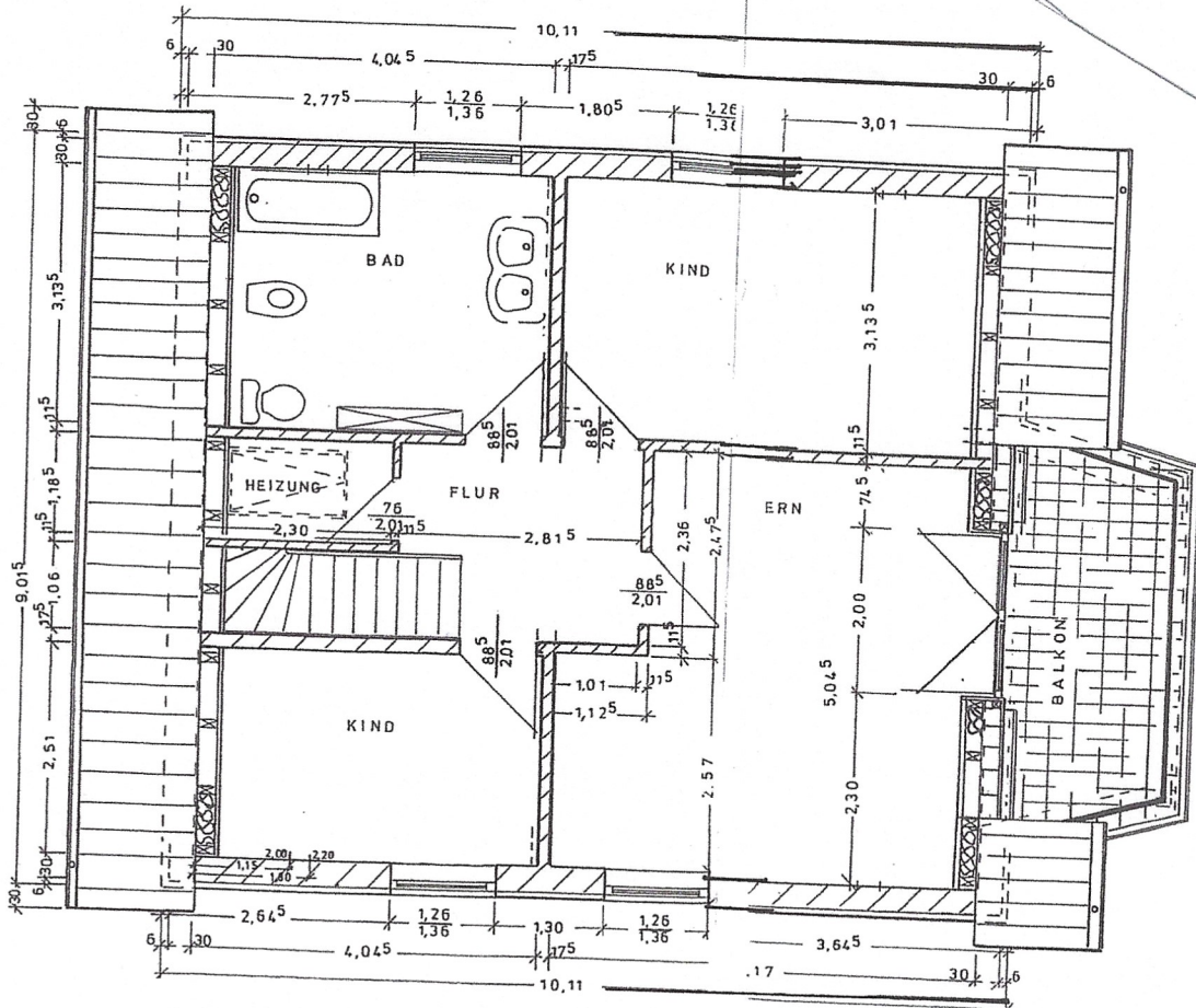
DACHGESCHOSSGRUNDRISS 1: 100
