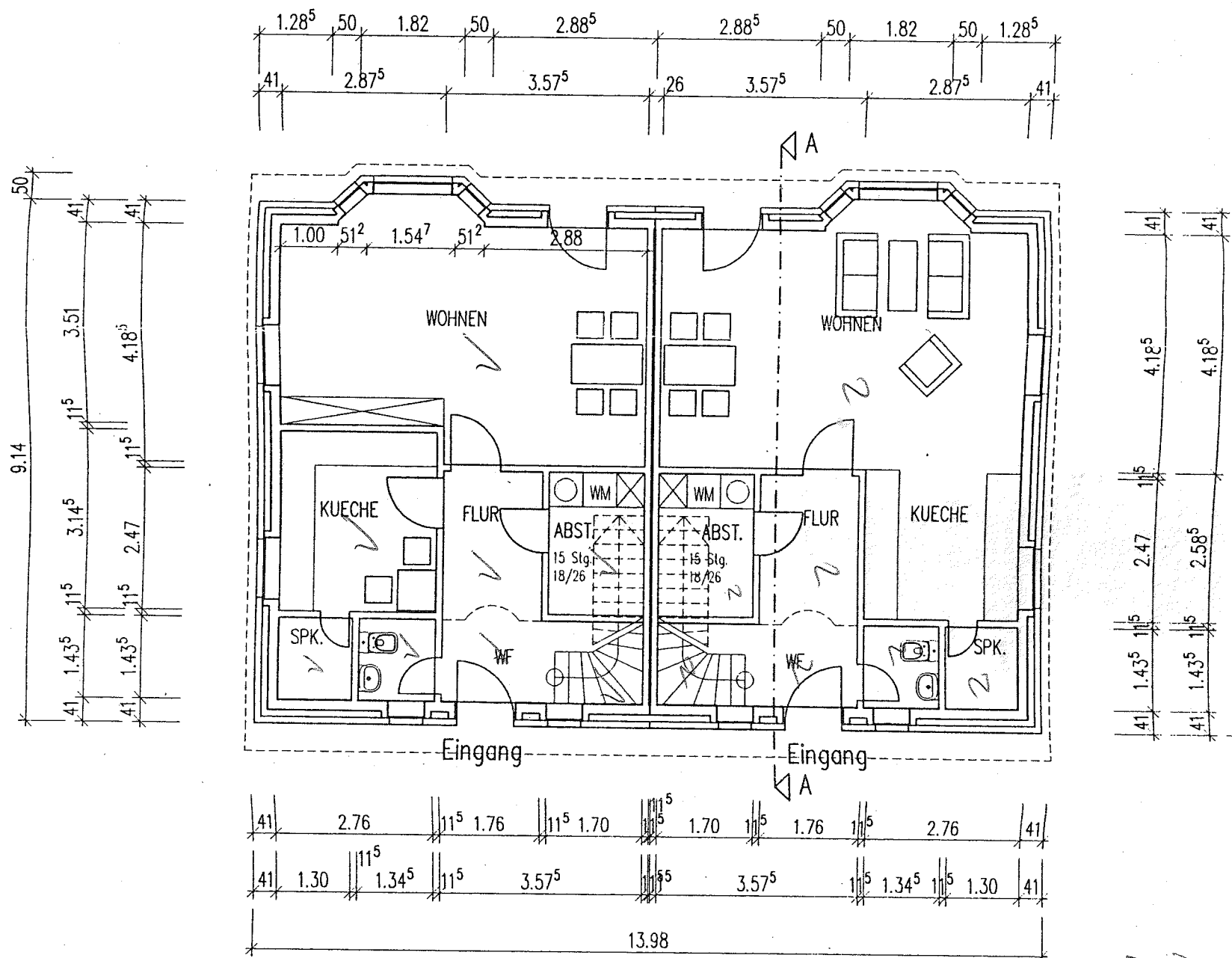
GRUNDRISS ERDGESCHOSS
