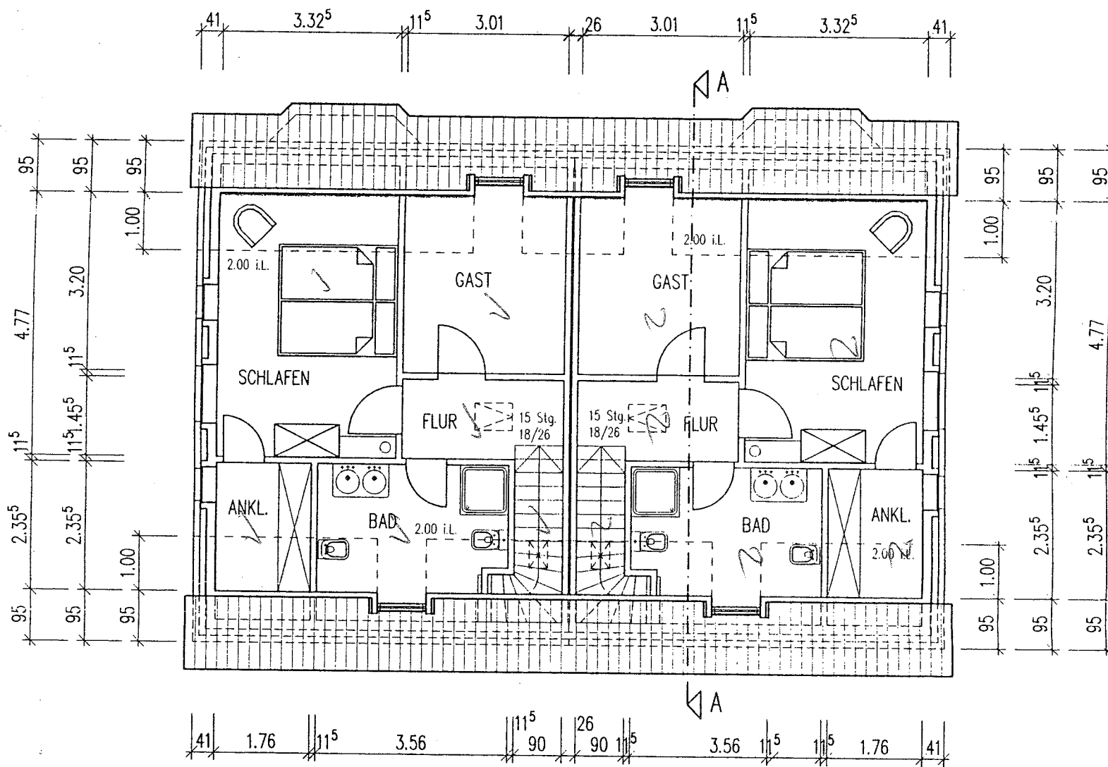
GRUNDRISS DACHGESCHOSS
