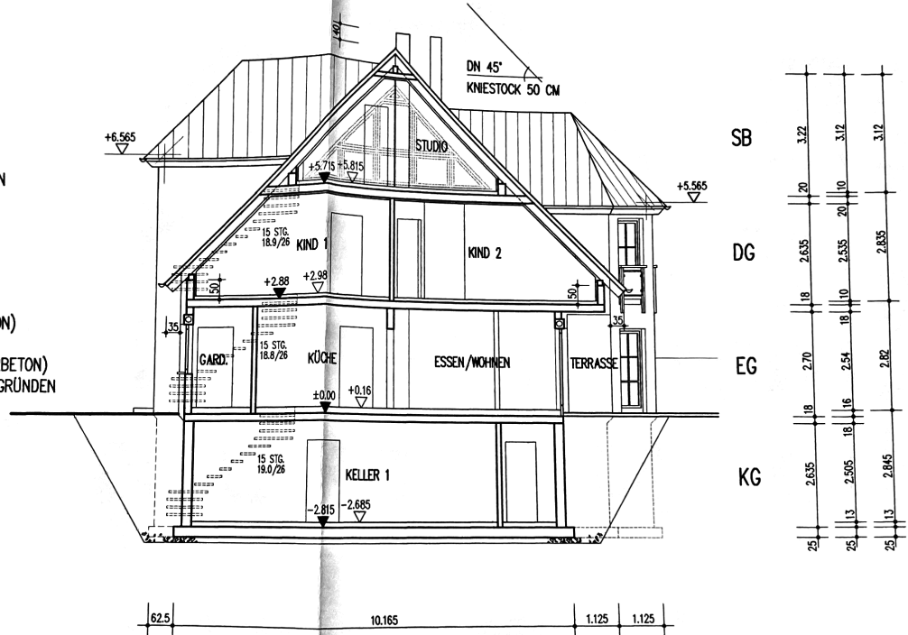
SNITT HAUS 1
