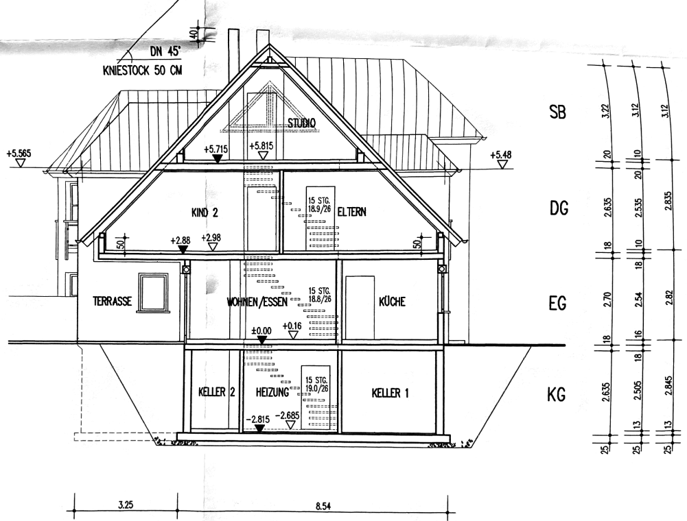
SCHNITT HAUS 2
