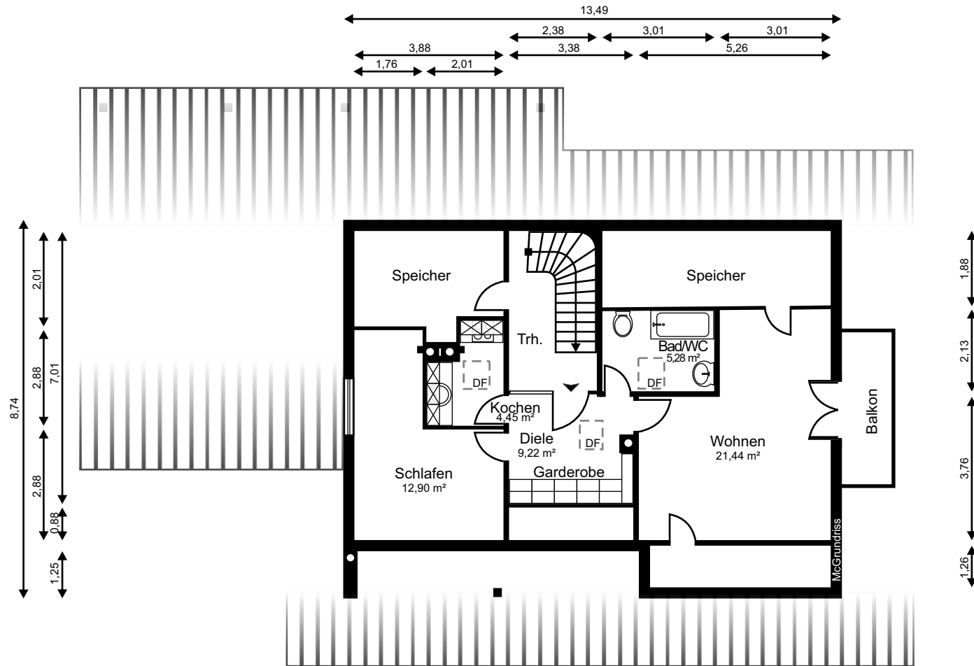
Dachgeschoss
