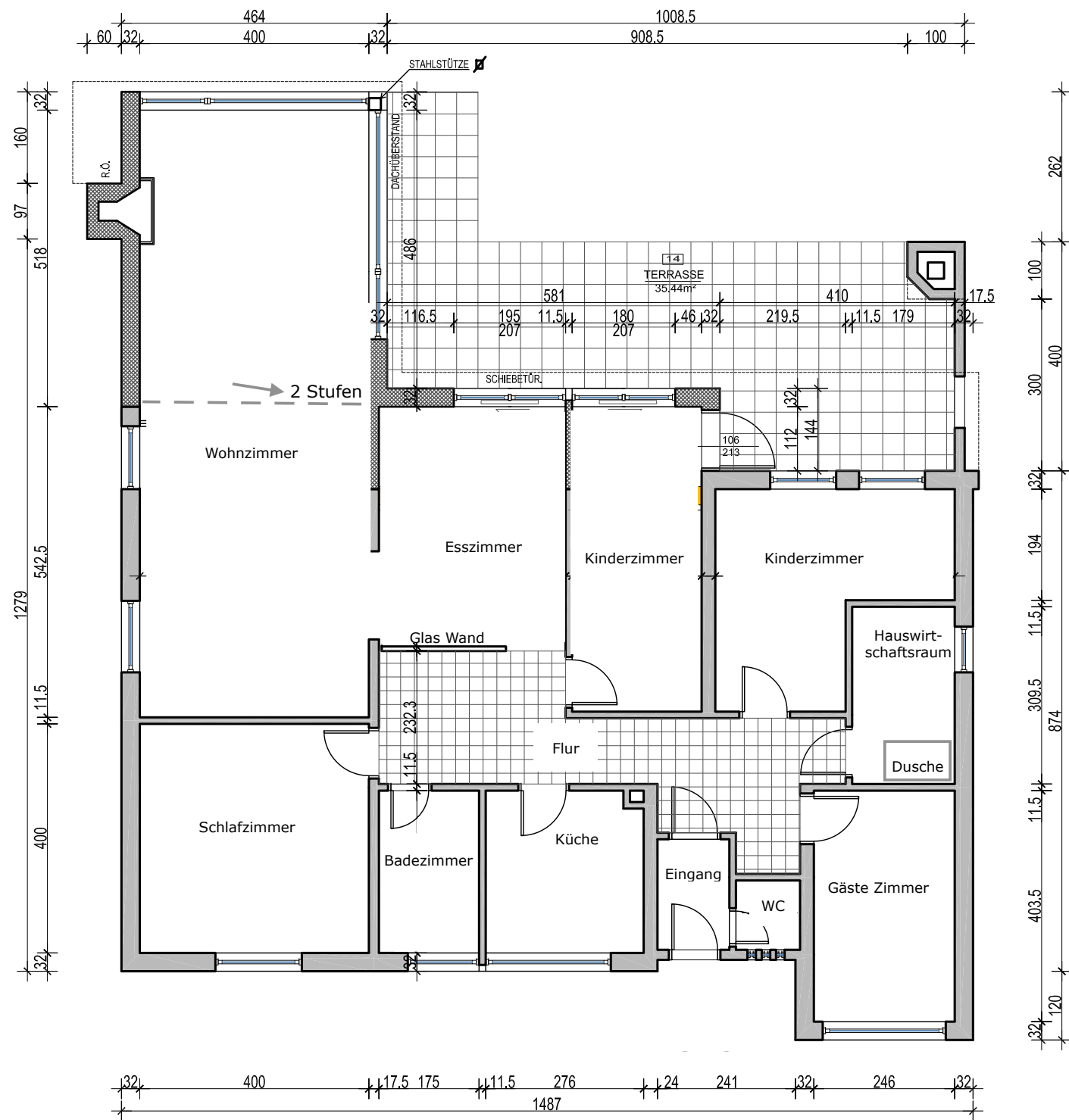
ERDGESCHOSS GRUNDRISS
