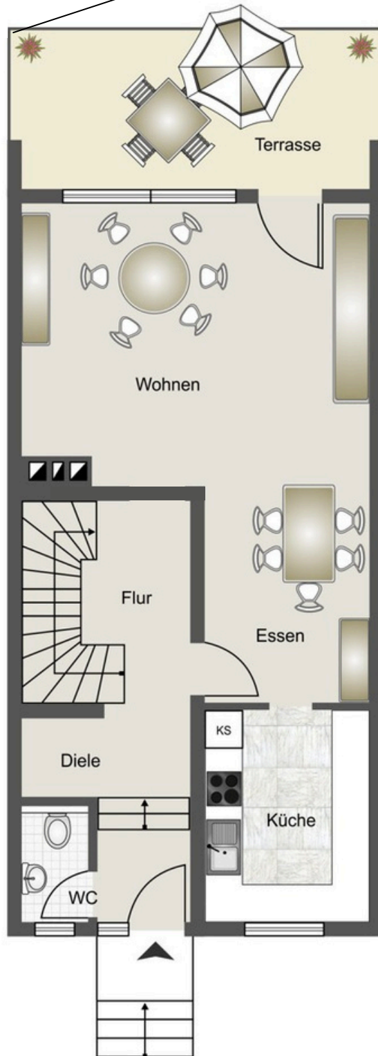
Erdgeschoss
