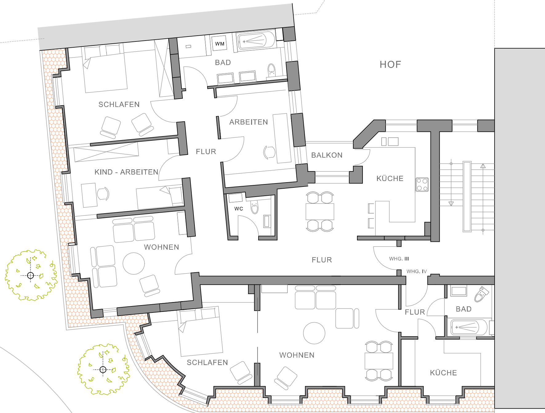
SEUMESTR.15 IN NÜRNBERG 2. OBERGESCHOSS
