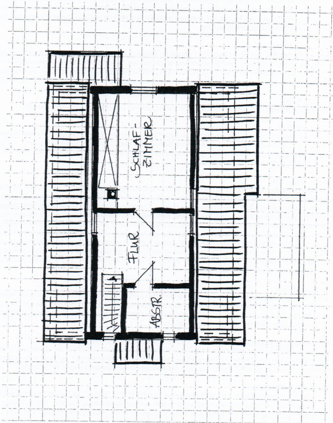
Dachgeschoss
