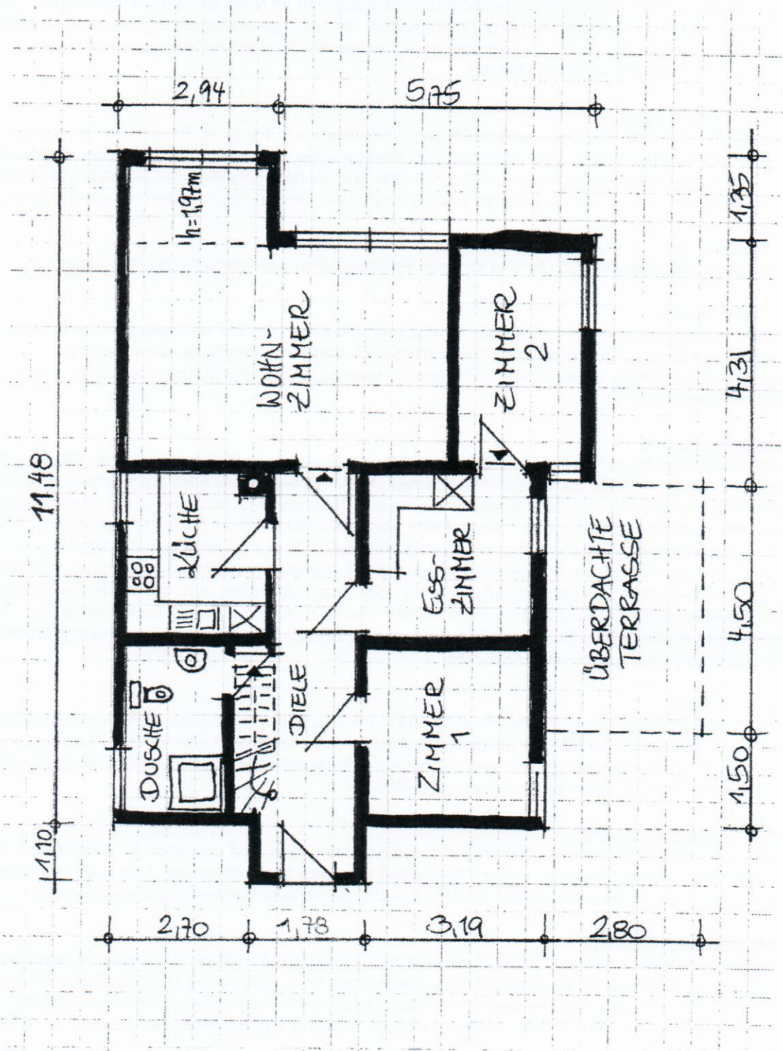
Erdgeschoss
