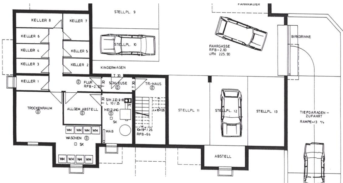
Kellerplan inkl. TG-Stellplätze
