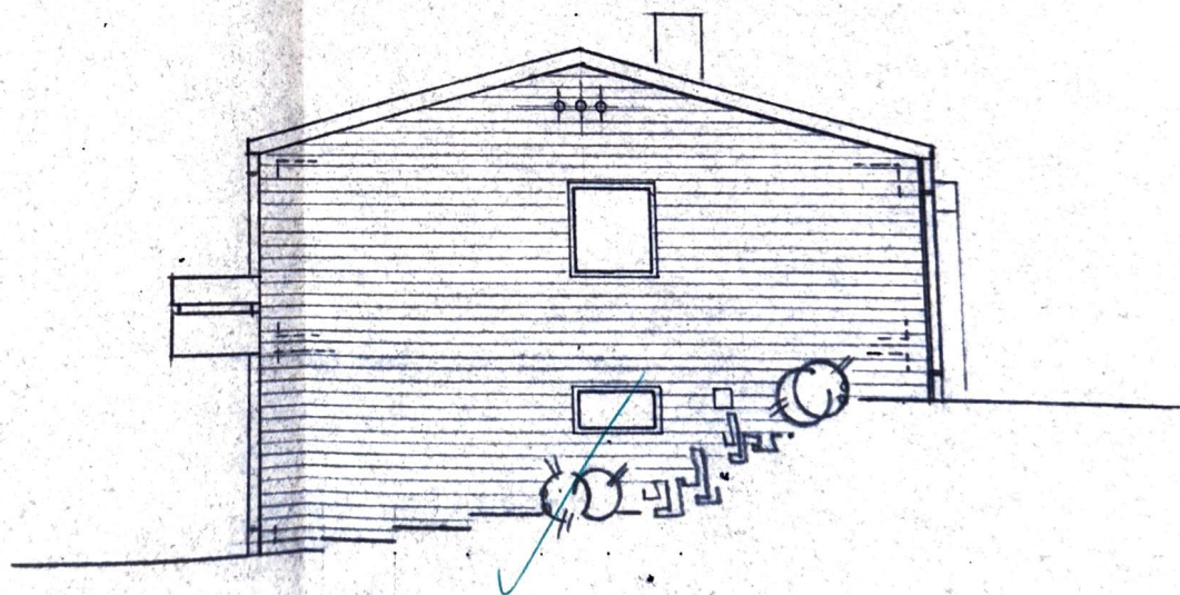
GIEBEL ANSICHT (RECHTS)
