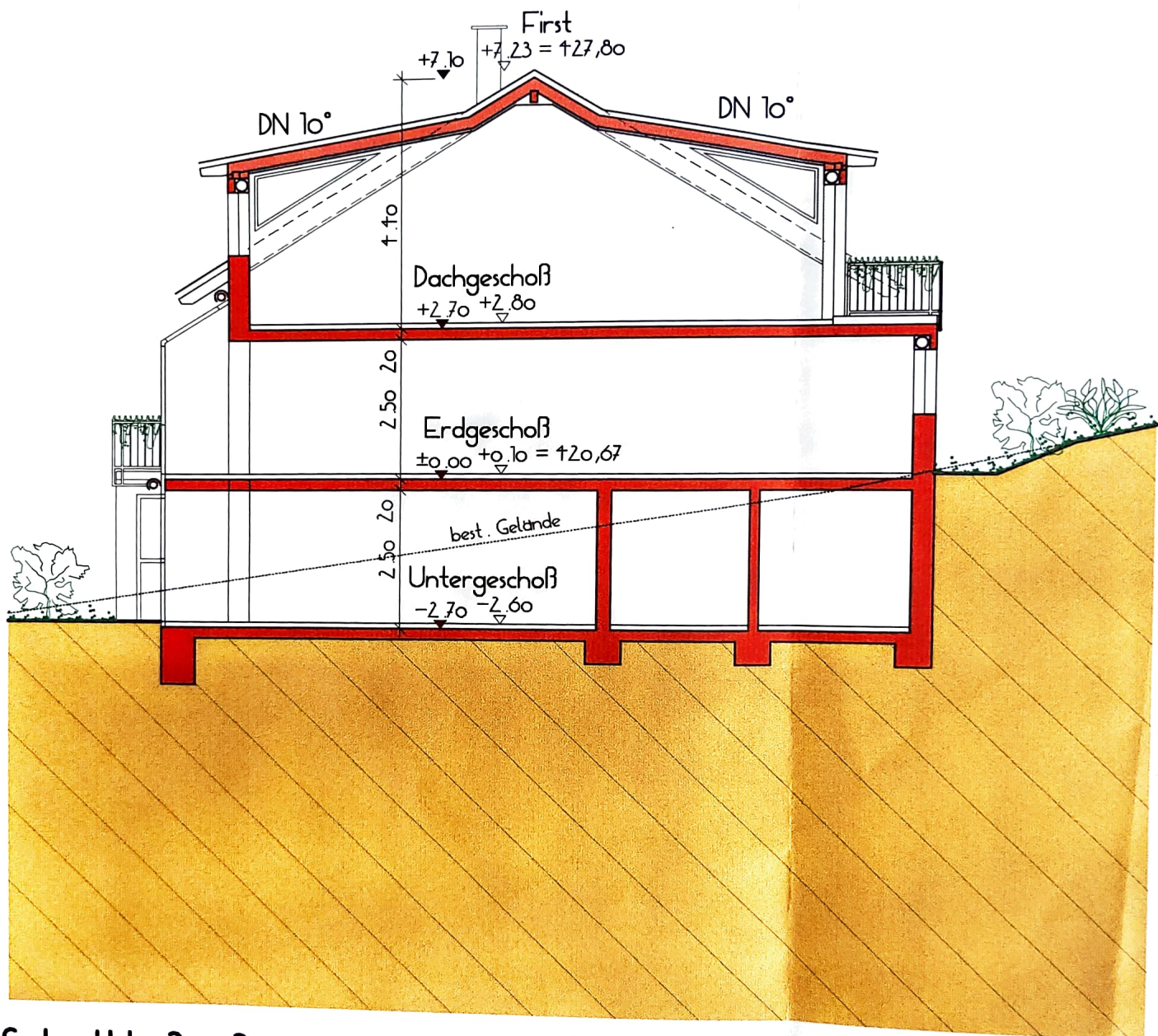
Schnitt 2-2
