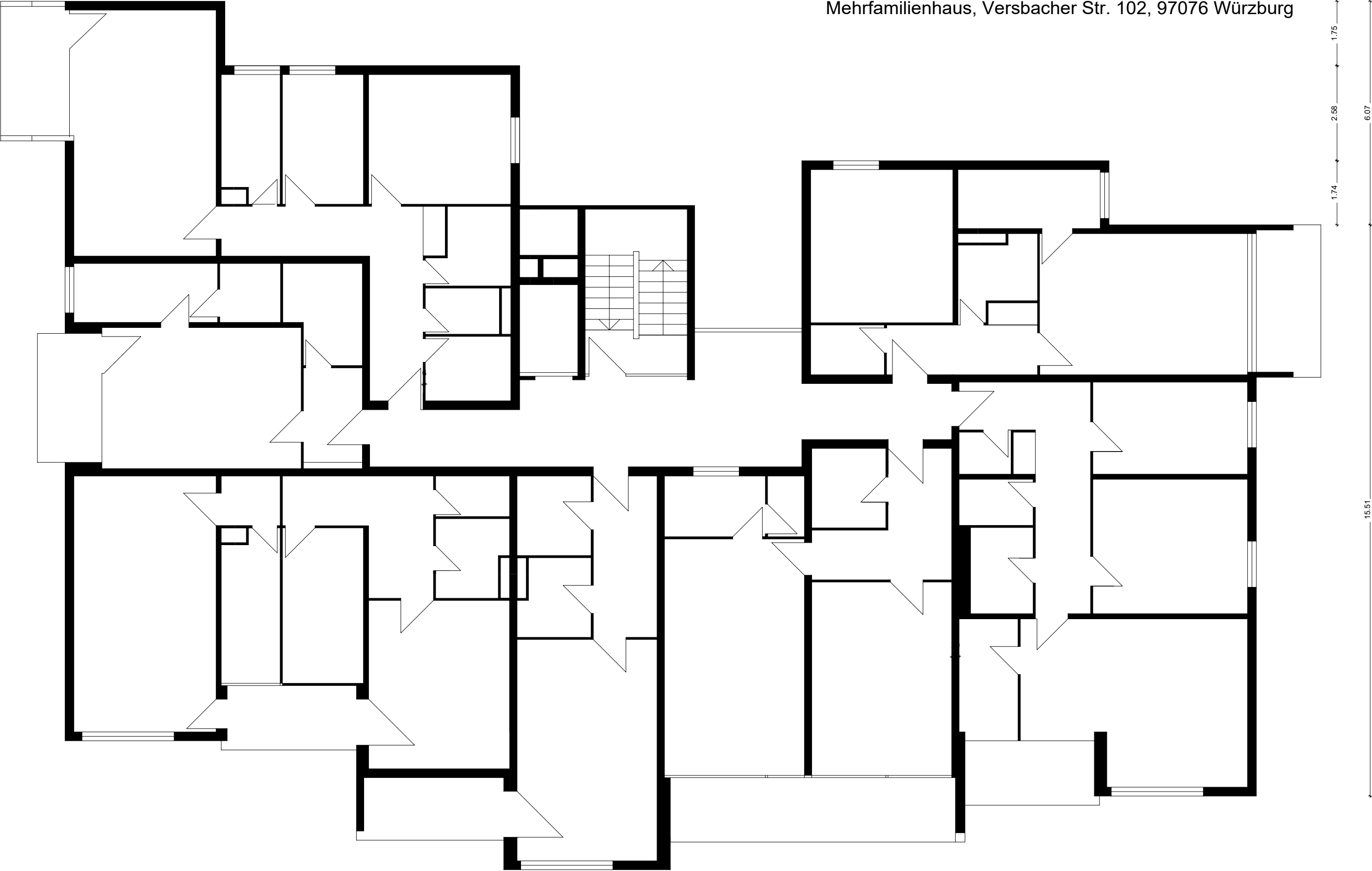
1.-5.Obergeschoss M. 1:100
