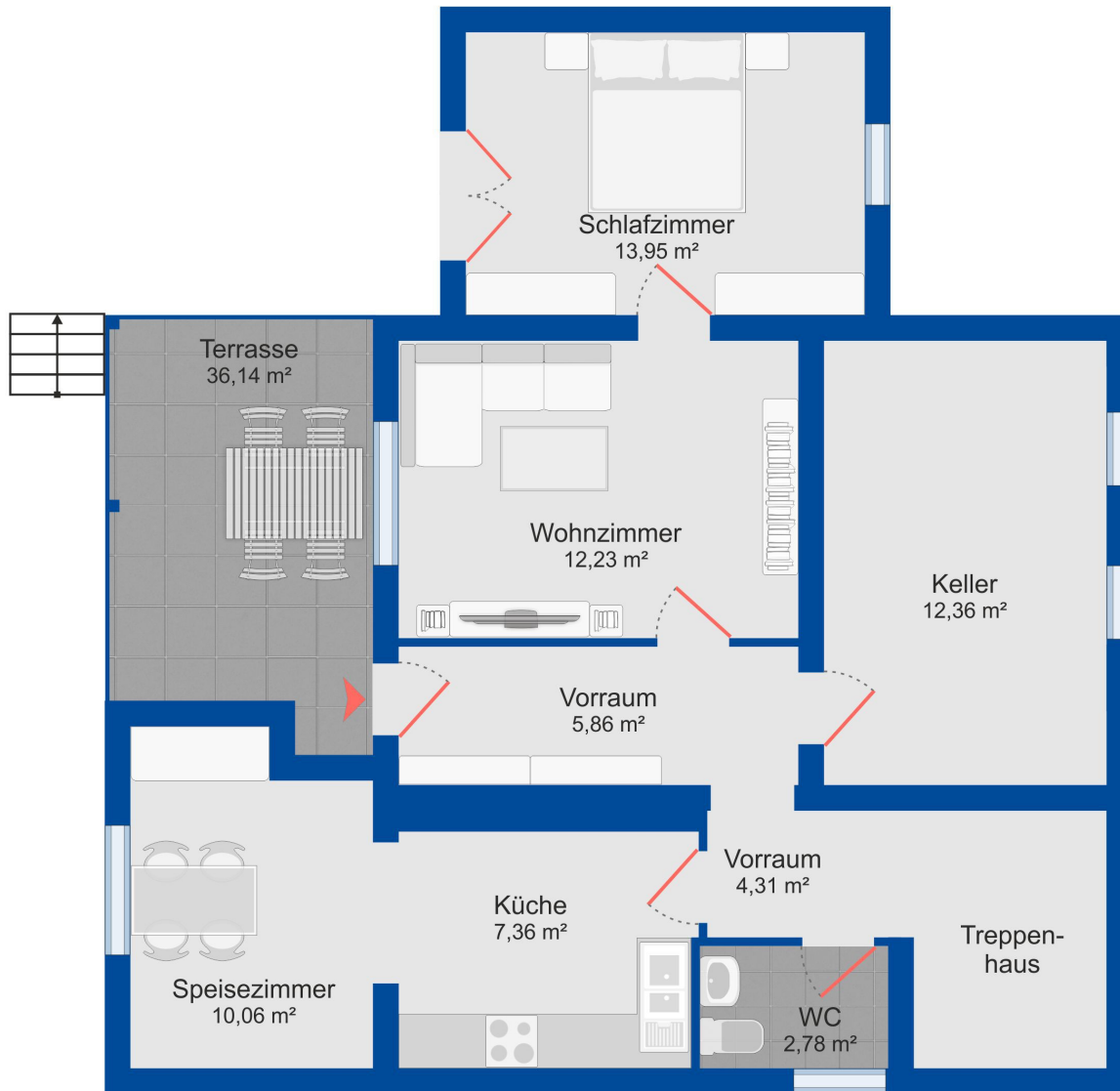
Untergeschoss
