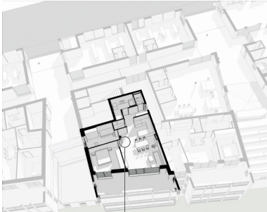
Top C04 - Haus C - EG
