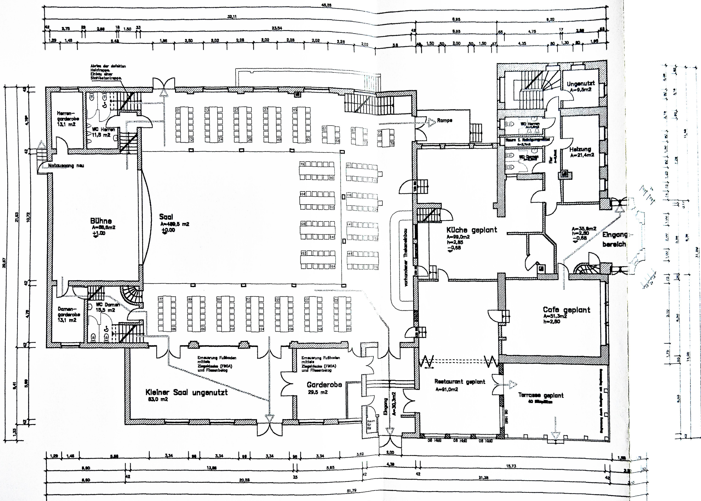
Grundriss Erdgeschoss
