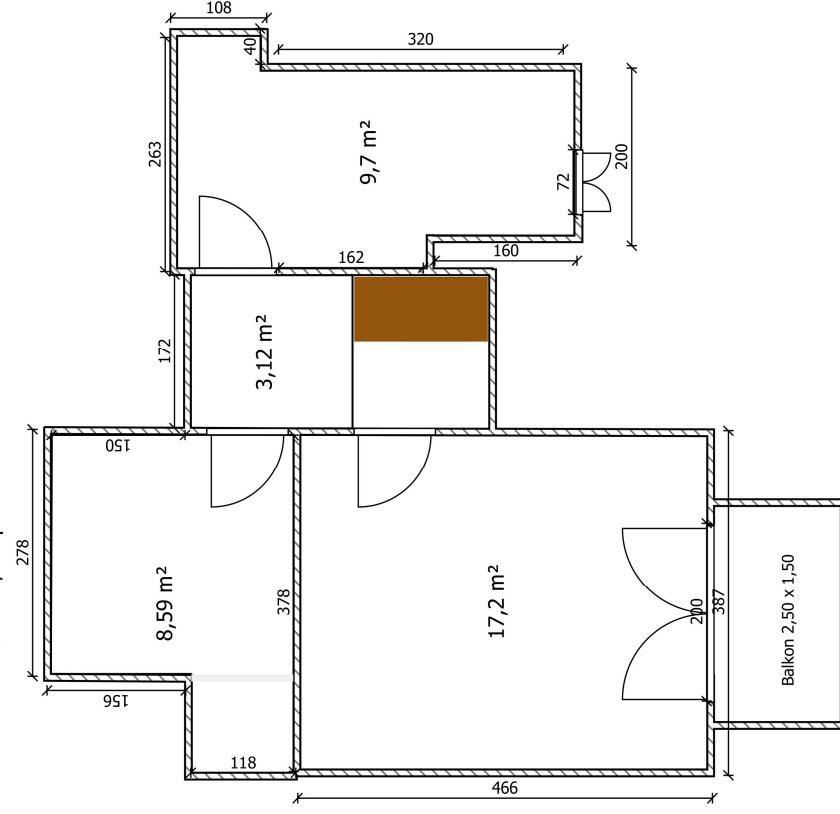
5. OG Gesamt 38,61 qm 2
