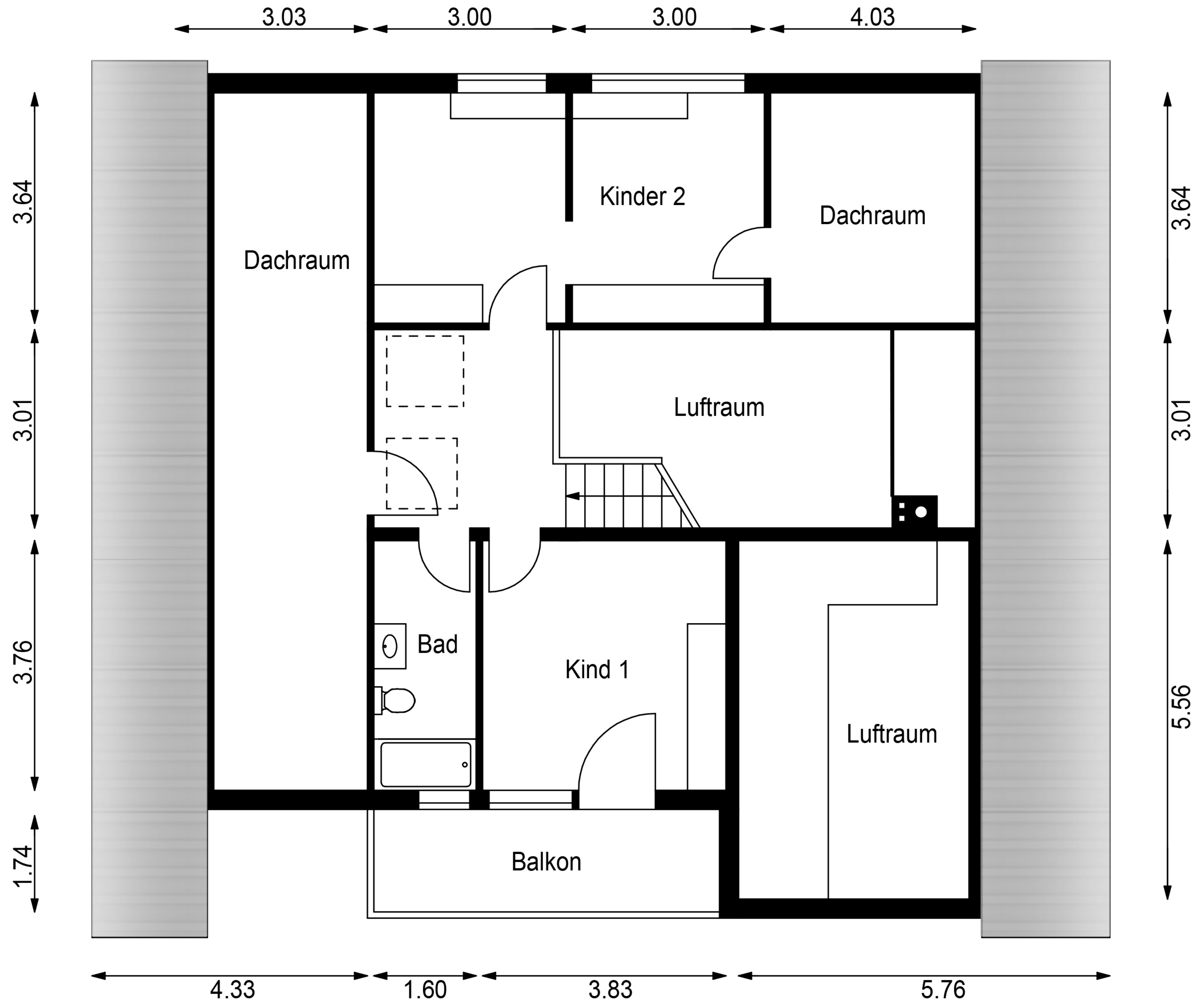
Dachgeschoss
