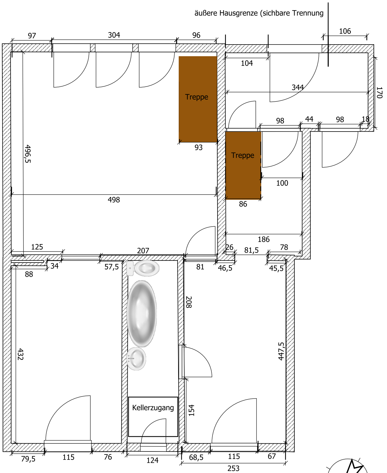
ERDGESCHOSS Maßstab 1:100
