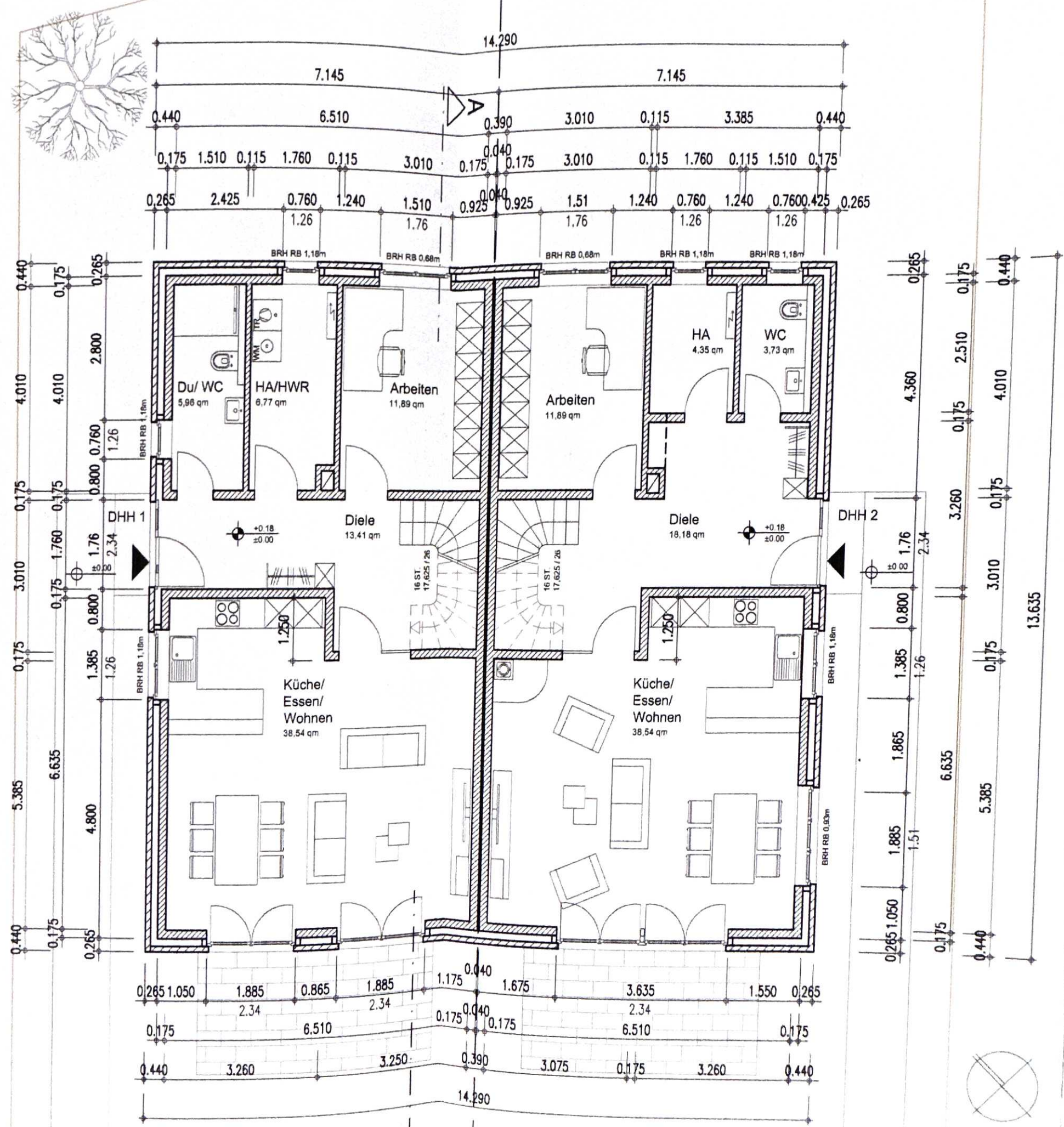
GRUNDRISS Erdgeschoss
