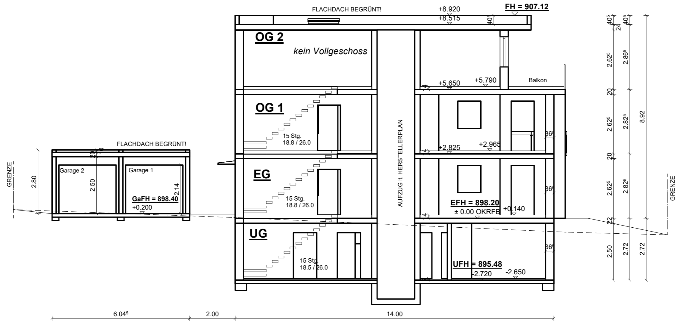
SCHNITT A-A
