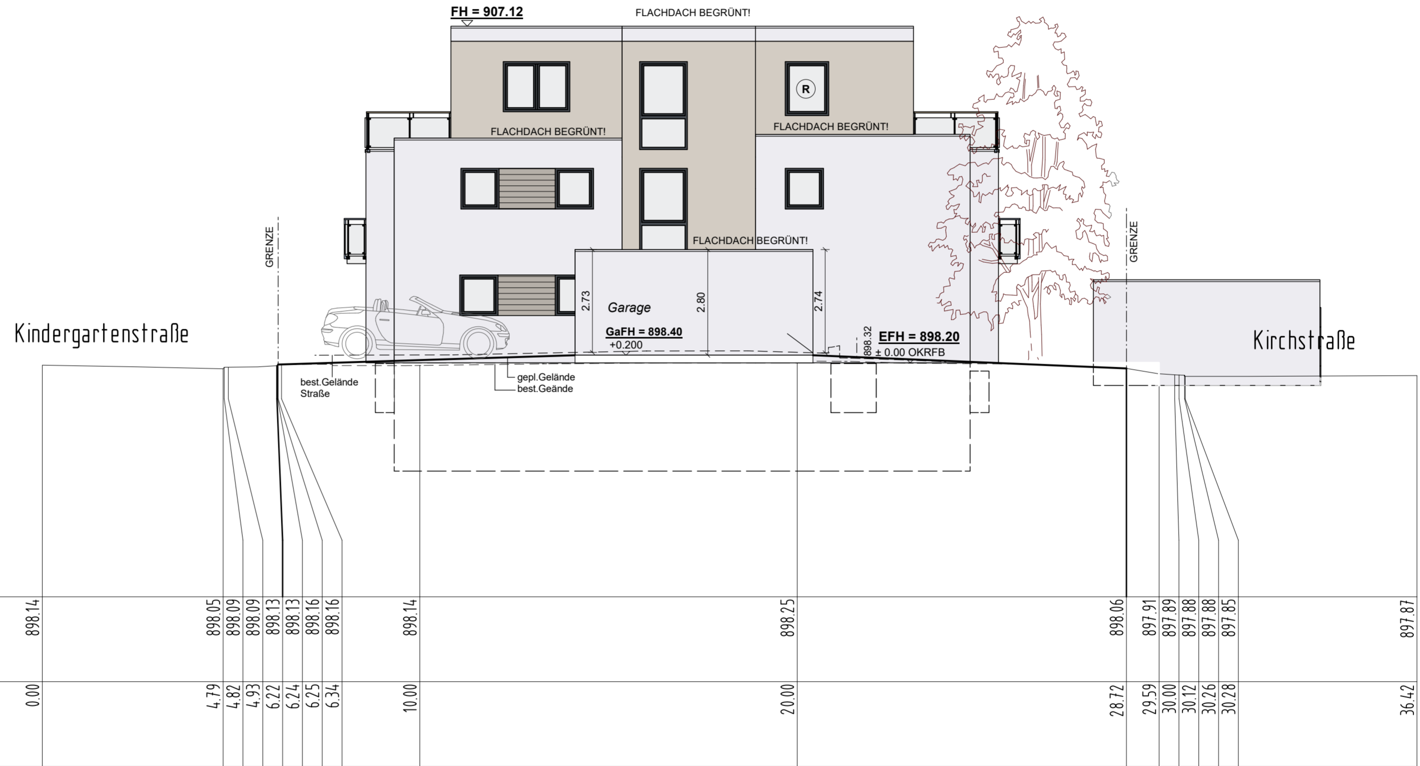
ANSICHT NORD
