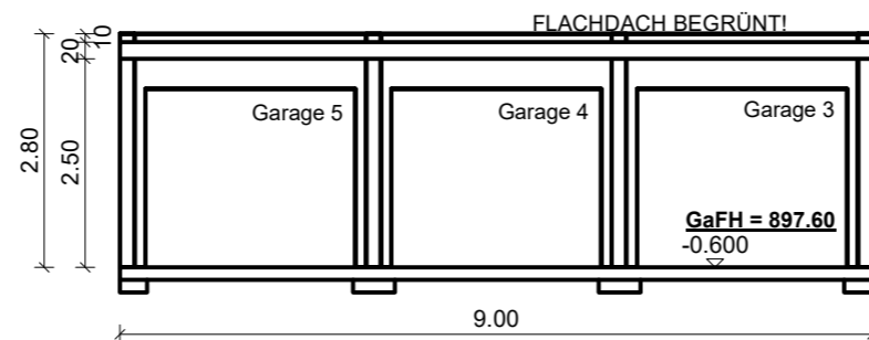
SCHNITT B - B
