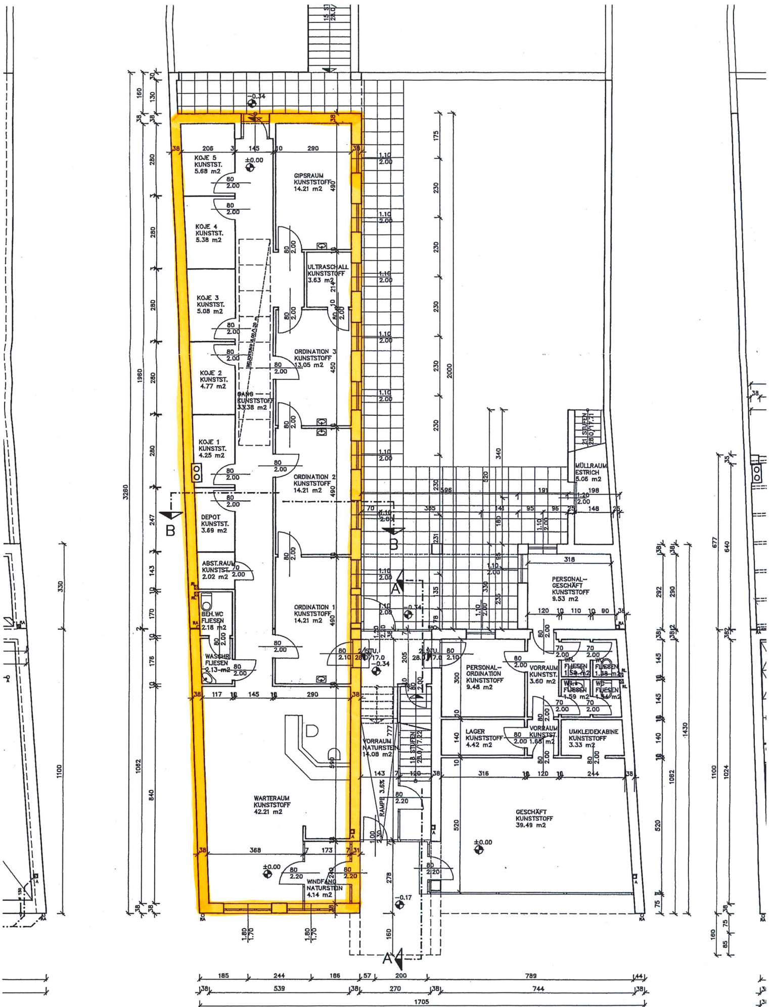
ERDGESCHOSS 1 : 100
