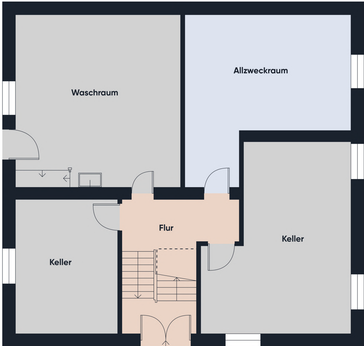
Grundrissplan ohne Maßstab KG
