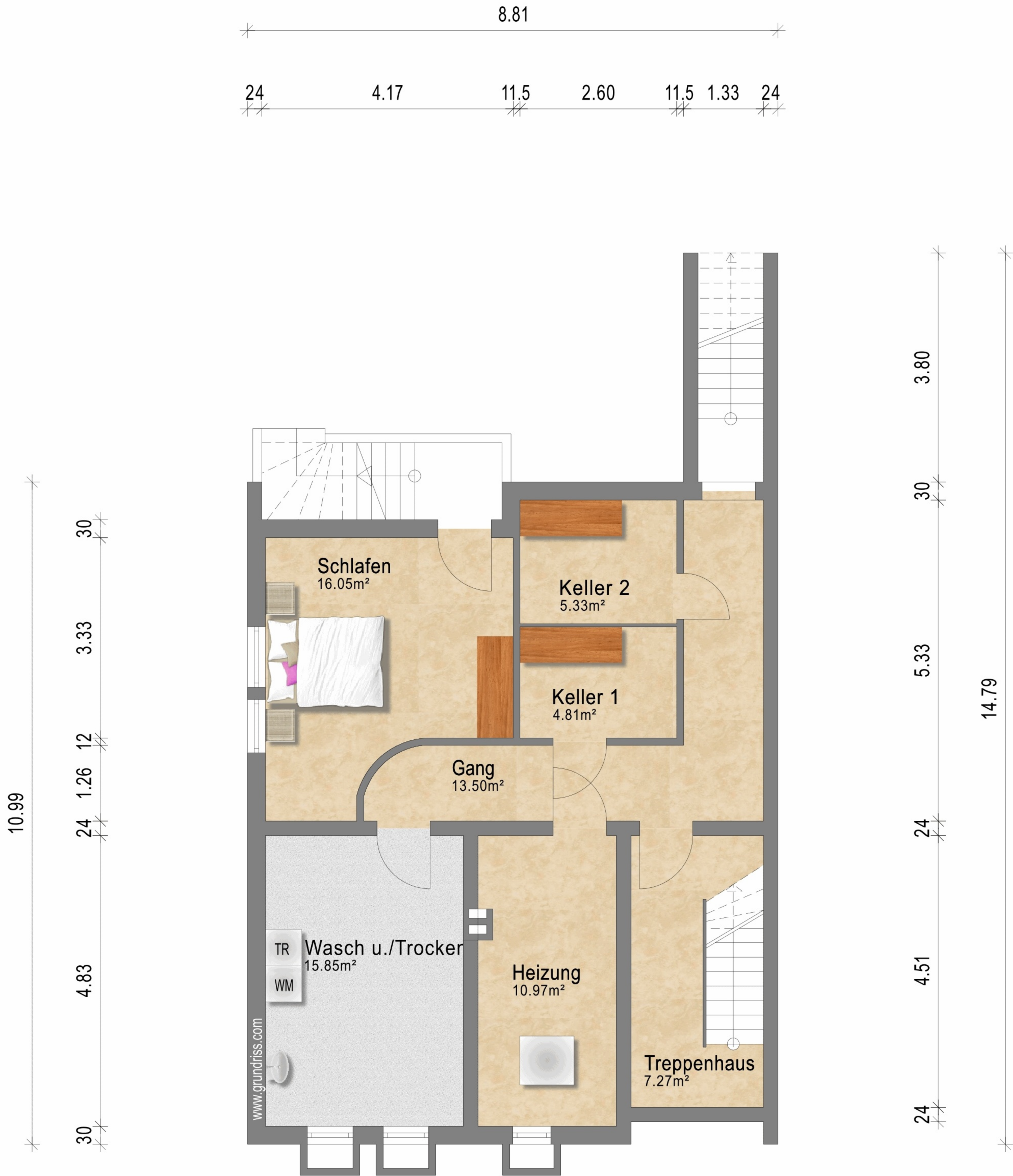
Kellergeschoss
