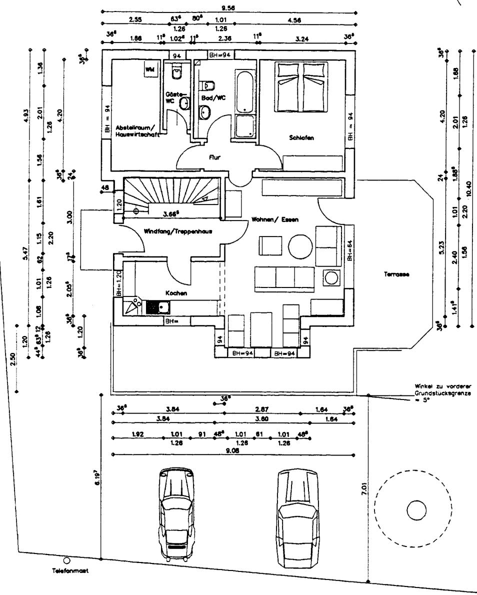
Lageplan und Grundriß Erdgeschoß
