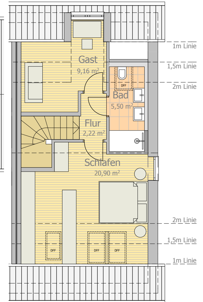
Dachgeschoss
