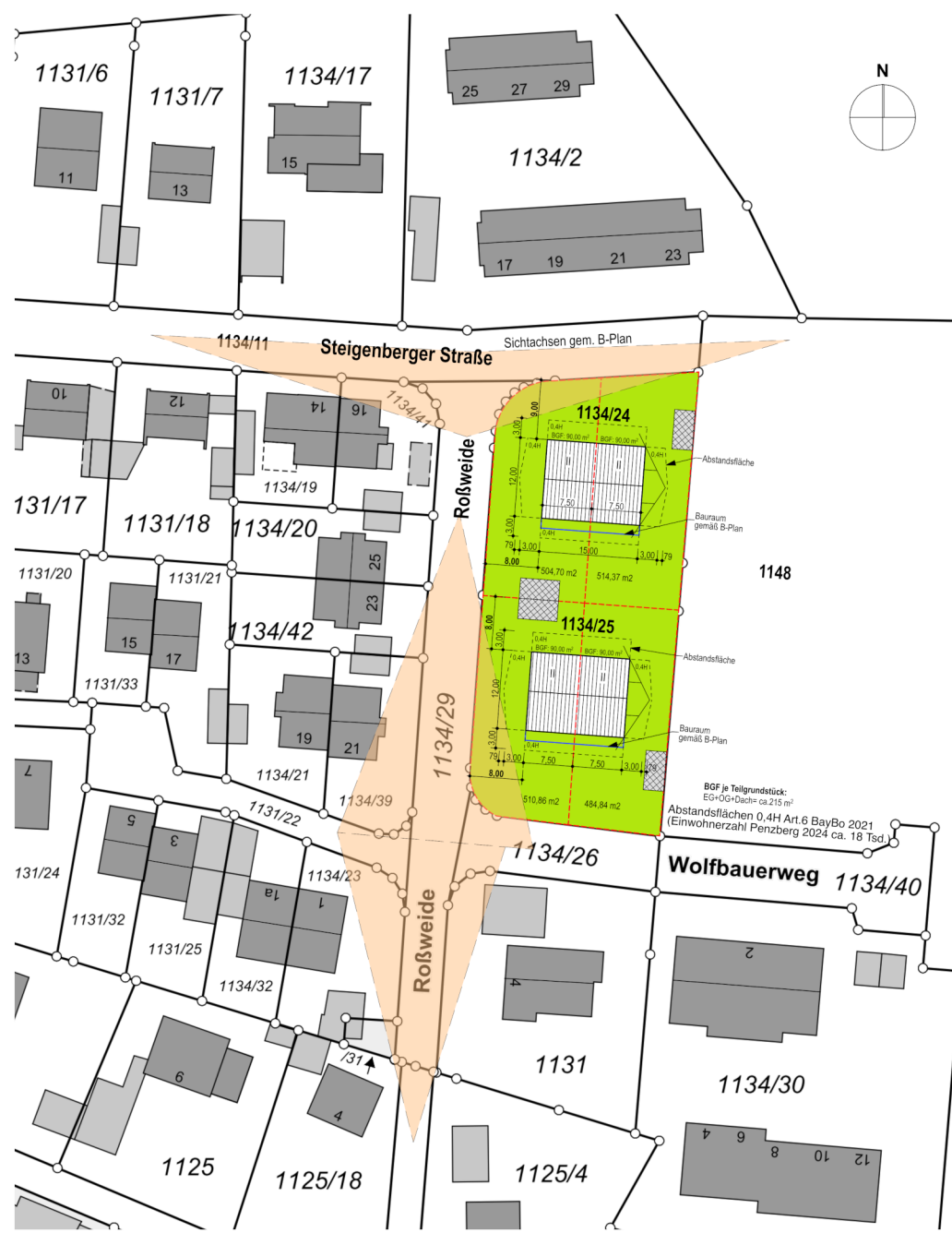
Lageplan M 1:500
