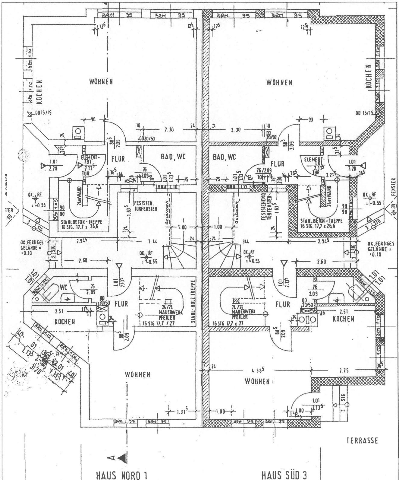
Grundriss Erdgeschoss
