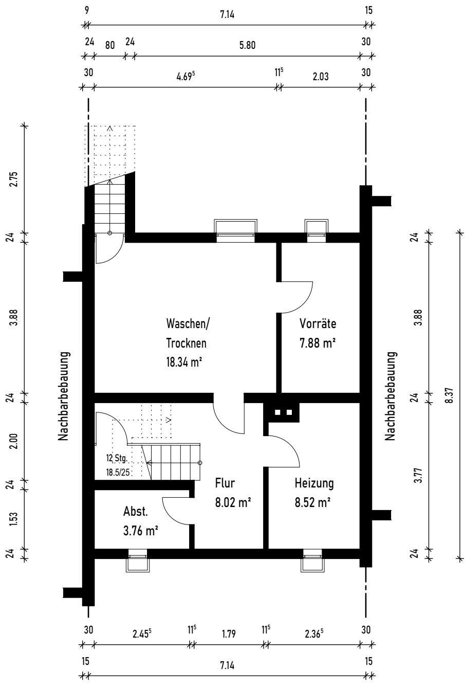
Kellergeschoss
