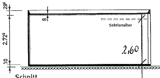
Schnitt
