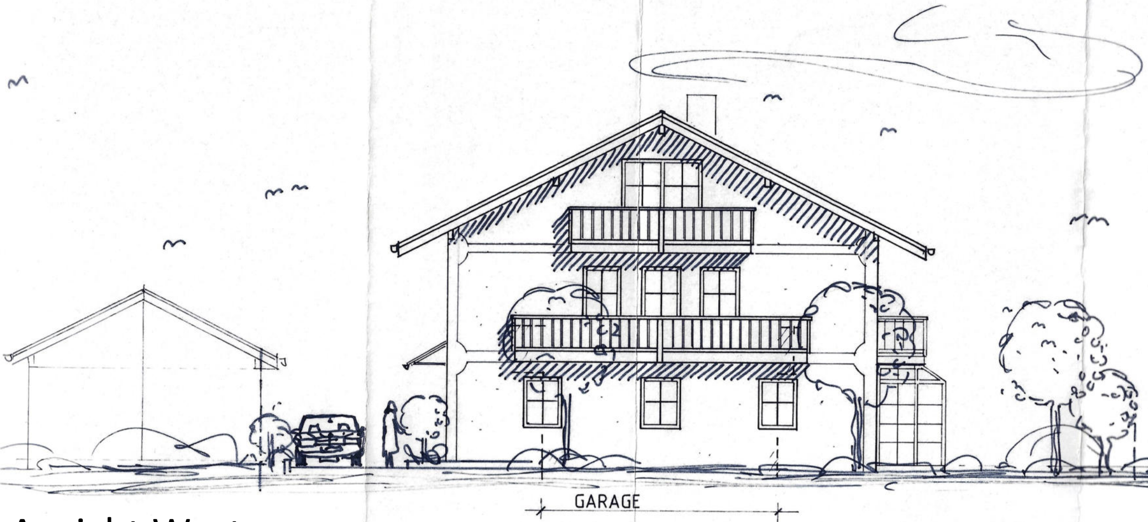
Ansicht West
