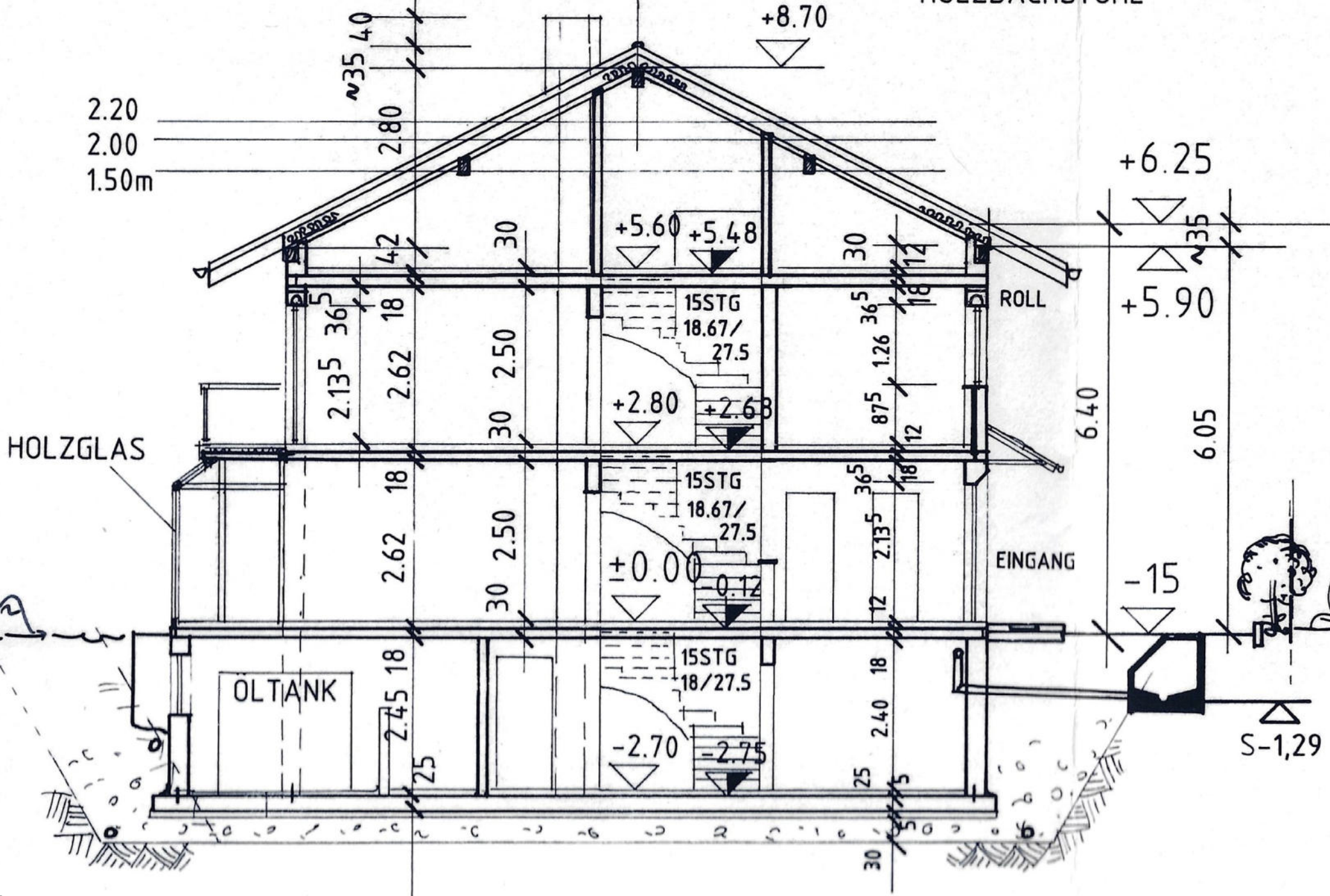
Schnitt A-A
