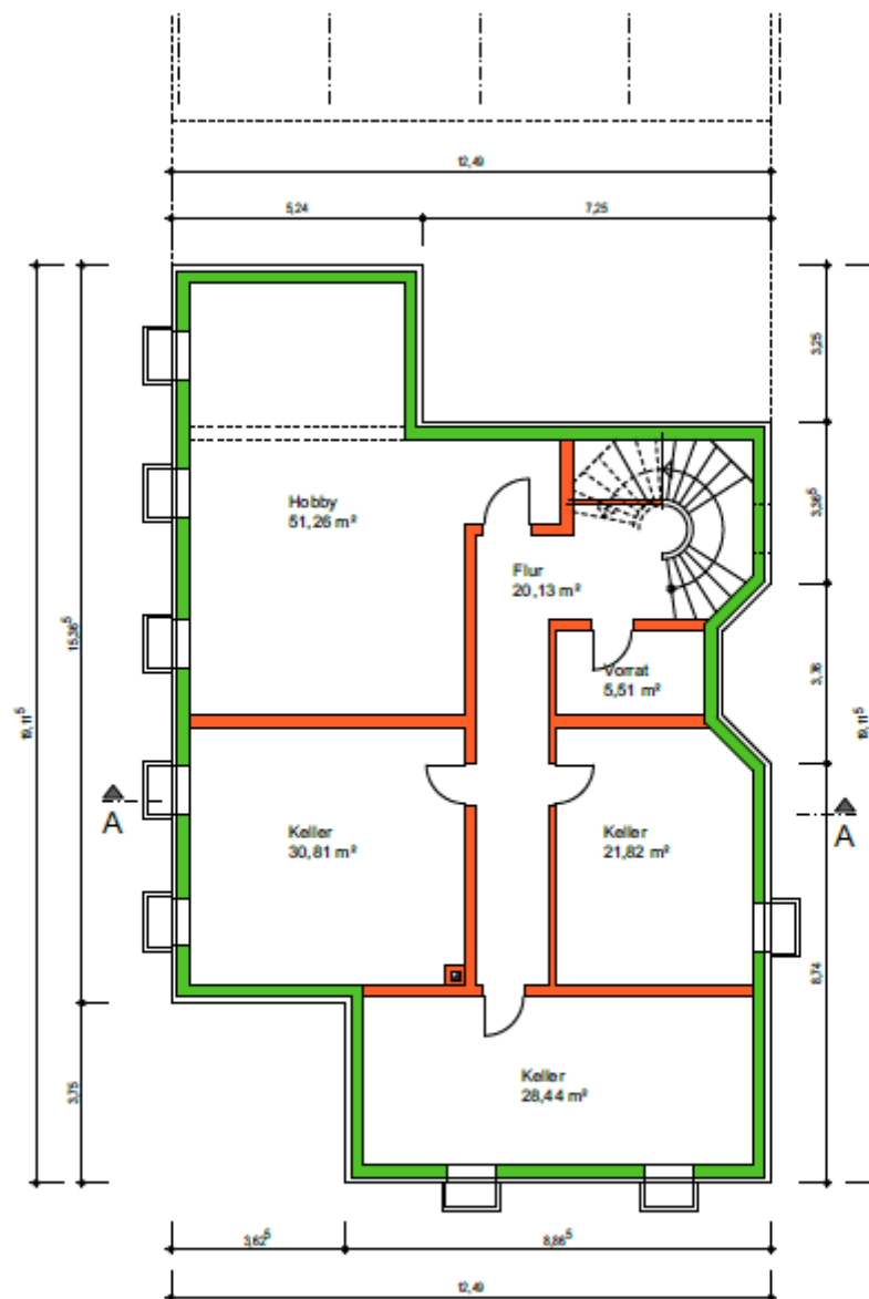
GRUNDRISS KELLERGECHOSS
