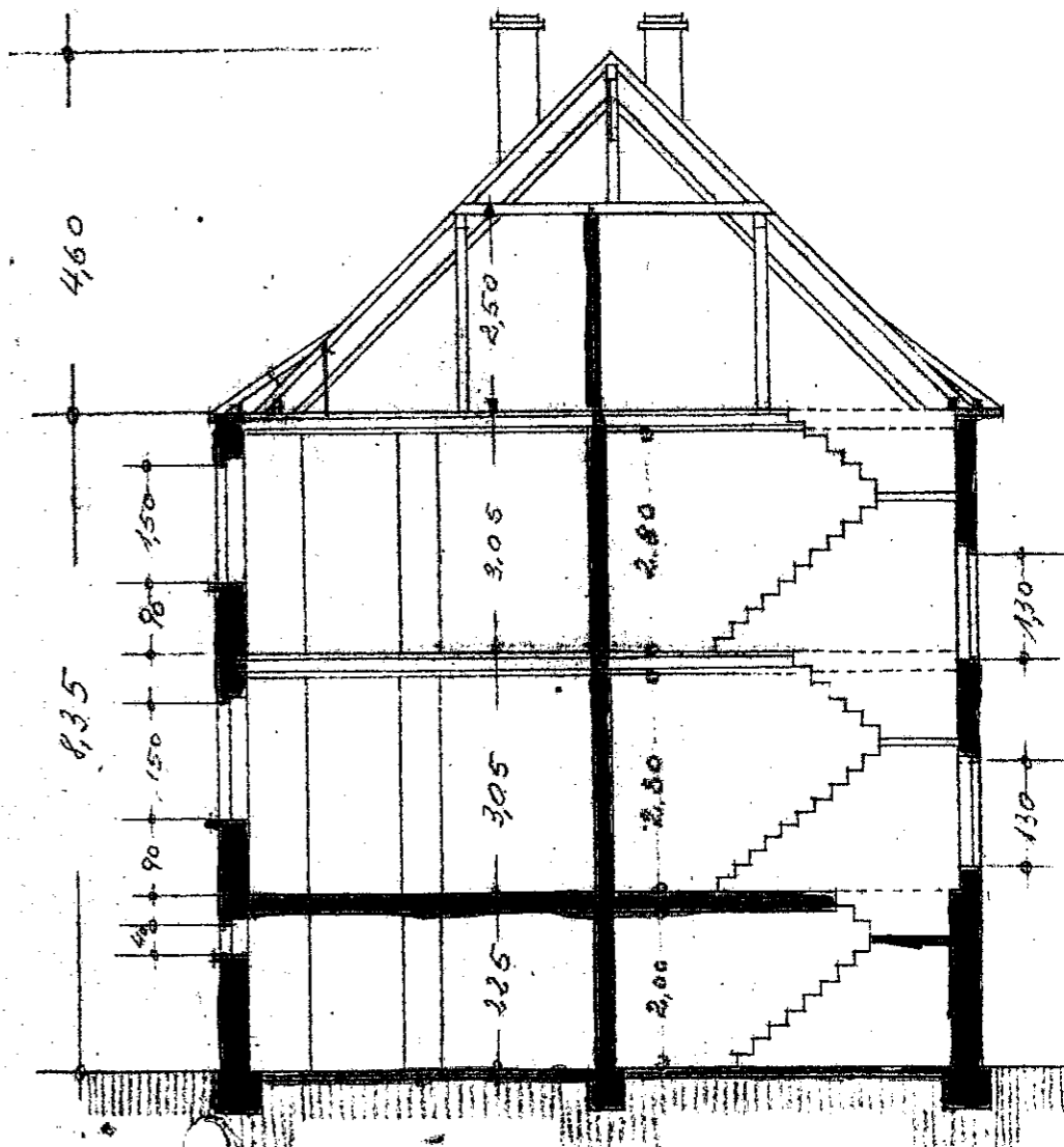
QUERSCHNITT
