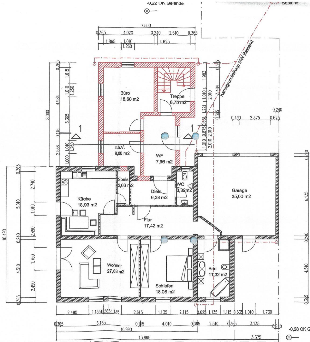
Grundriss Erdgeschoss
