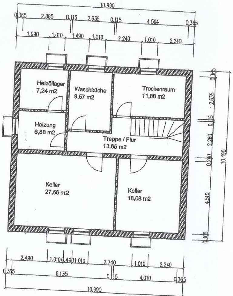
Grundriss Kellergeschoss
