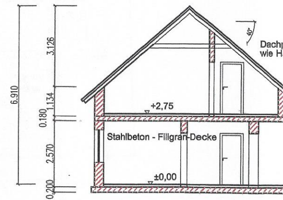
Schnitt 1-1
