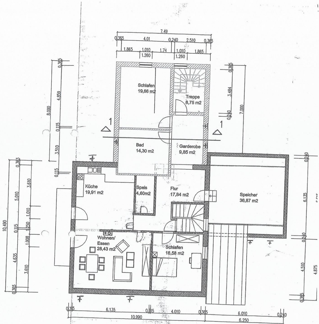
Grundriss Obergeschoss
