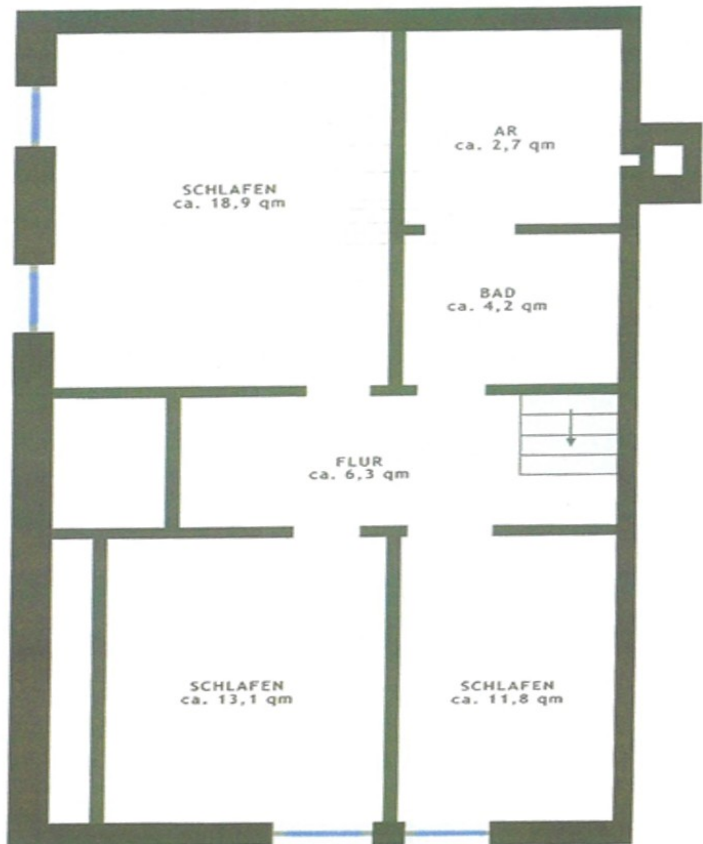
Grundriss Dachgeschoss - nicht maßstabsgetreu
