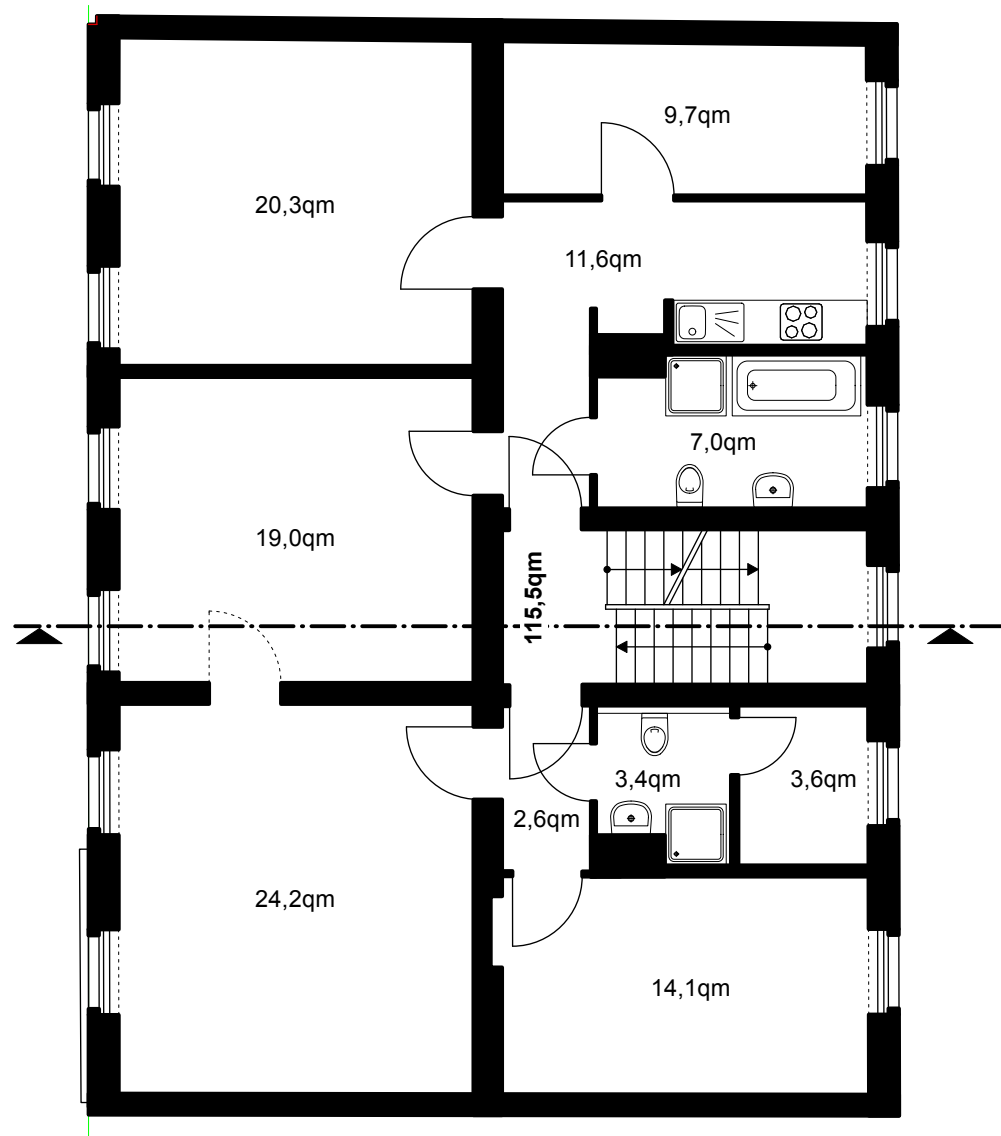
1.Obergeschoß
