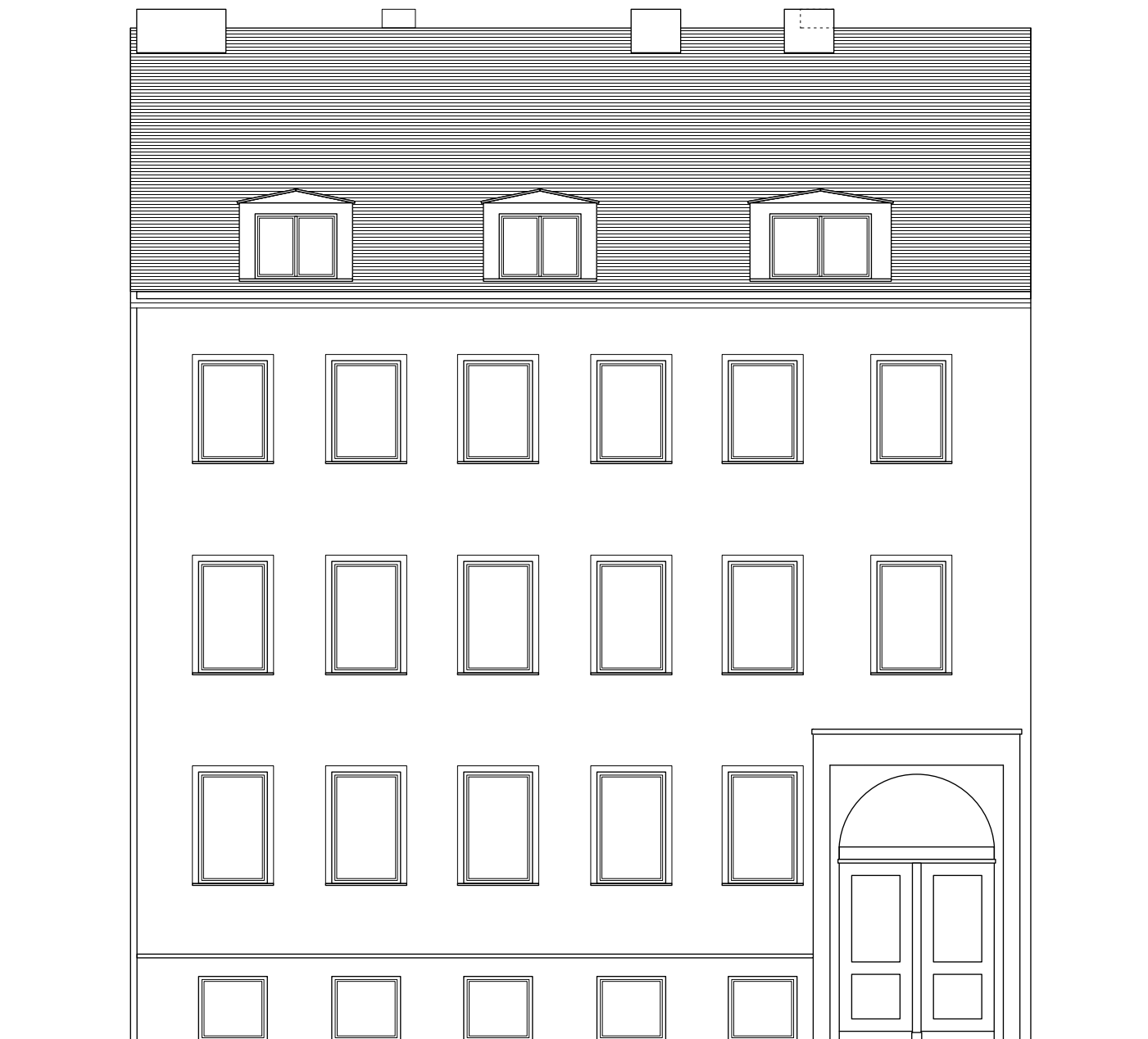
Straßenansicht
