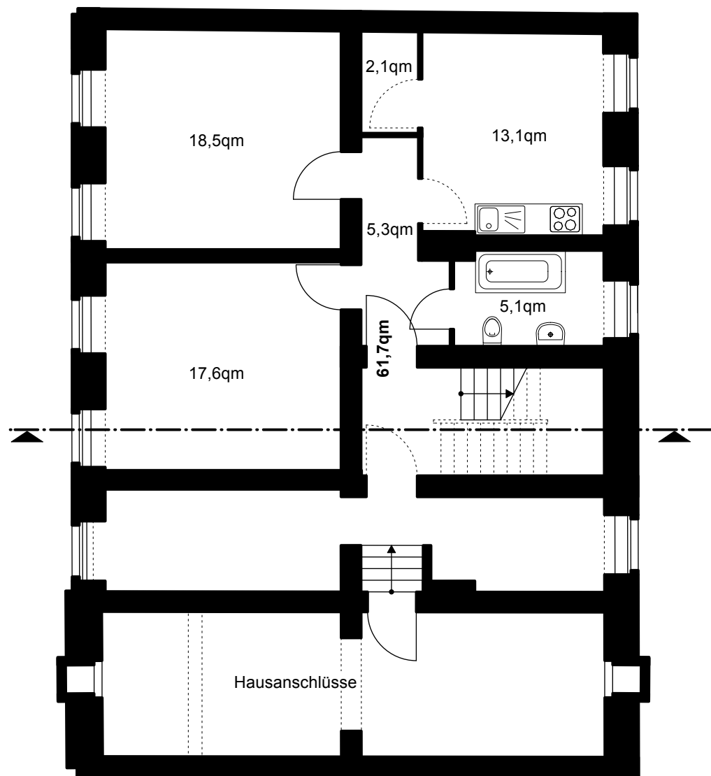
Kellergeschoß
