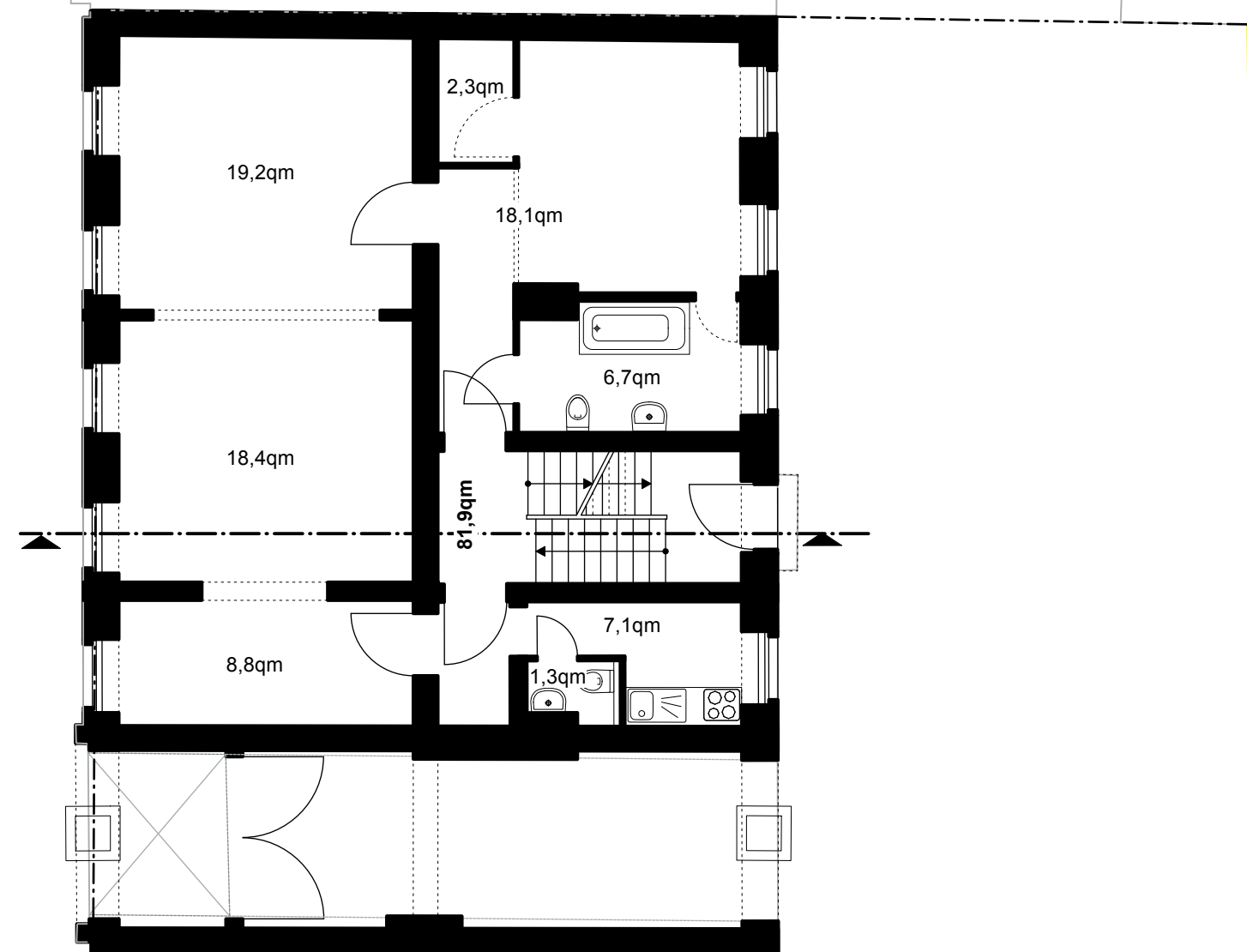
Hochparterre / Erdgeschoß
