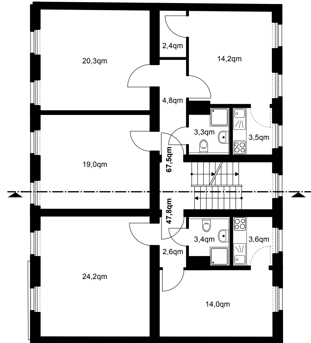
2.Obergeschoß
