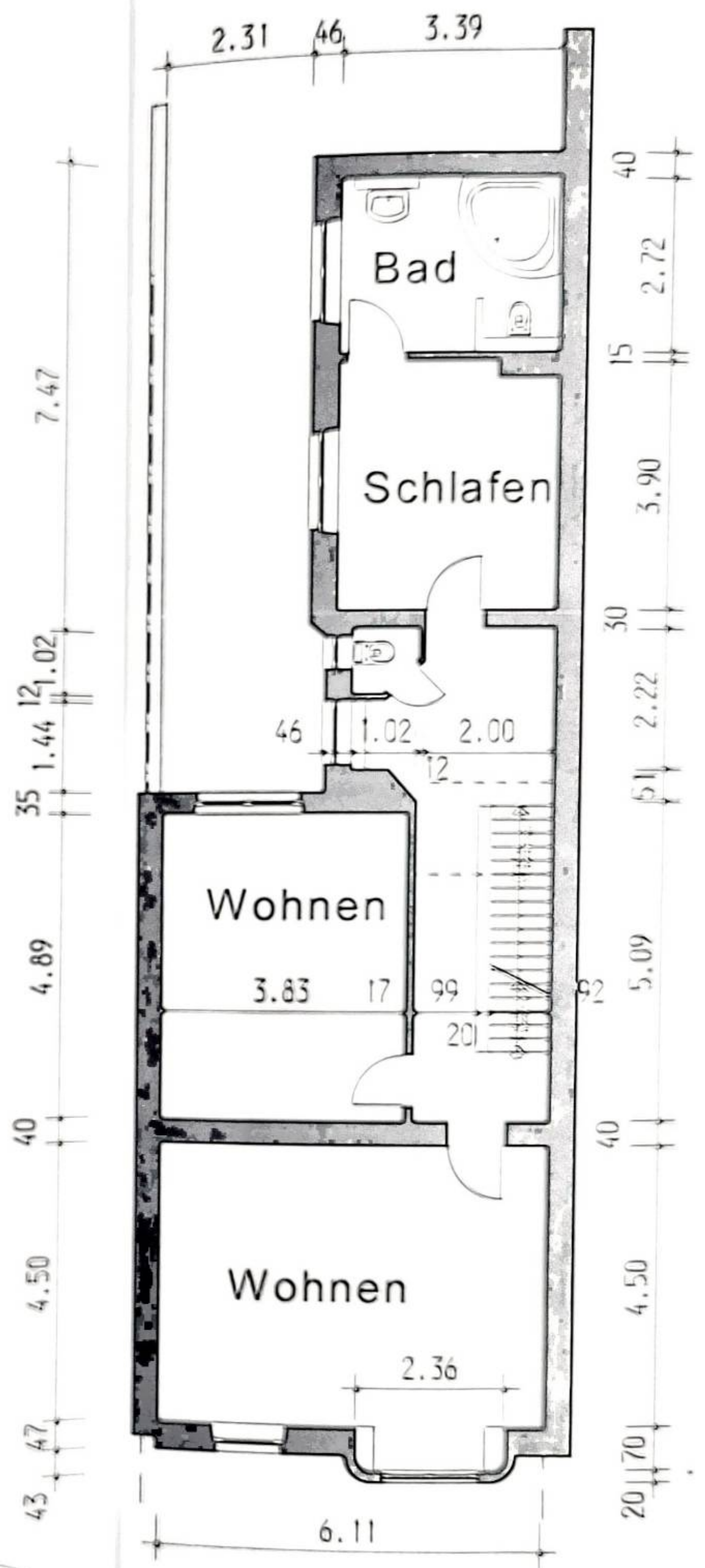
1. OBERGESCHOSS Ebene +3.39 m
