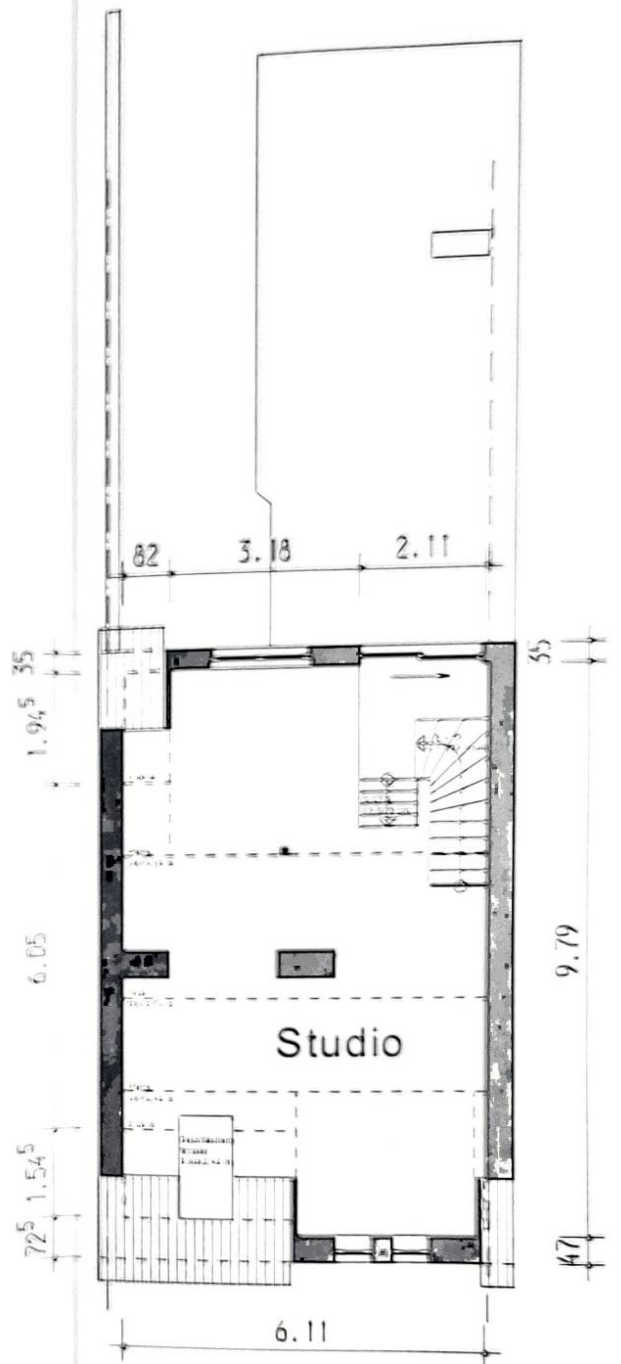
DACHGESCHOSS Ebene +9.62 m
