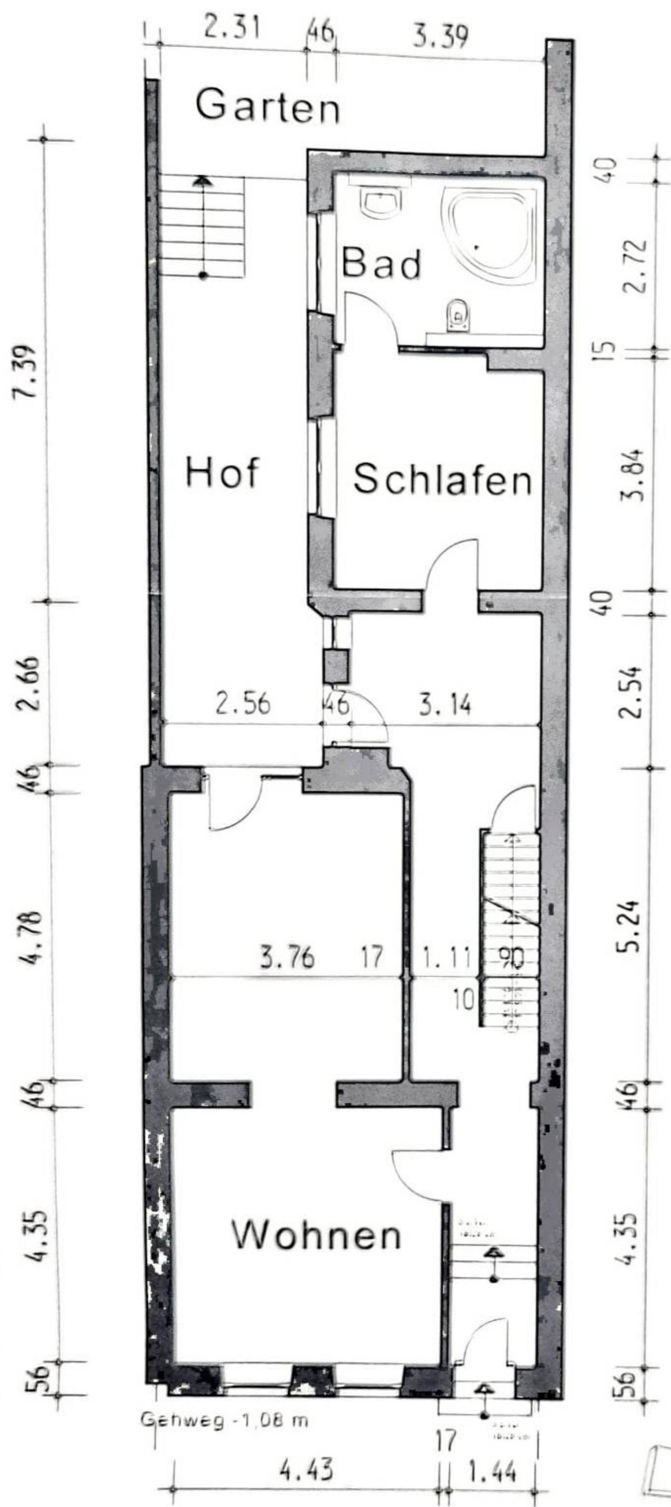
ERDGESCHOSS Ebene 0.00 m
