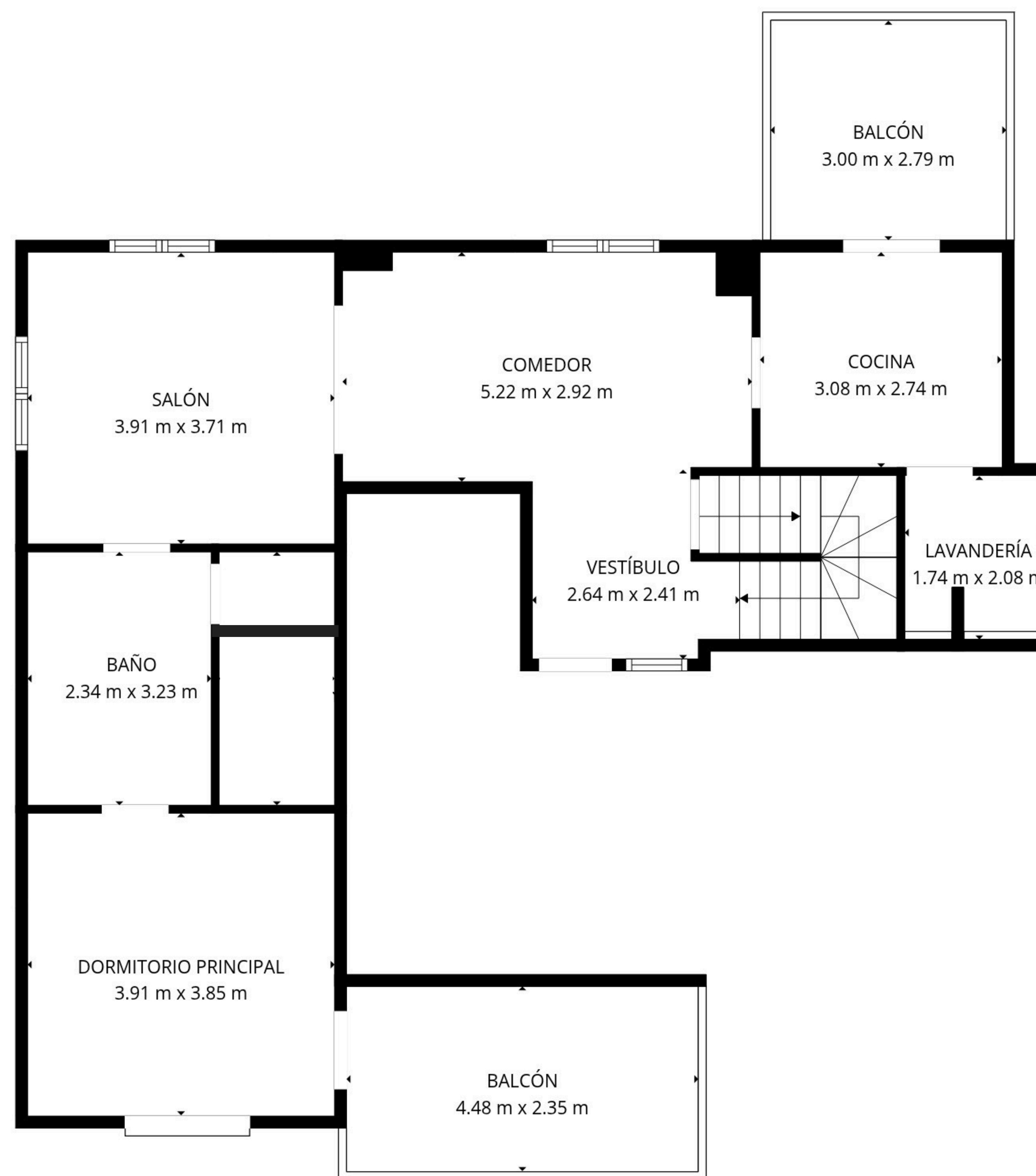
2. PLANTA
