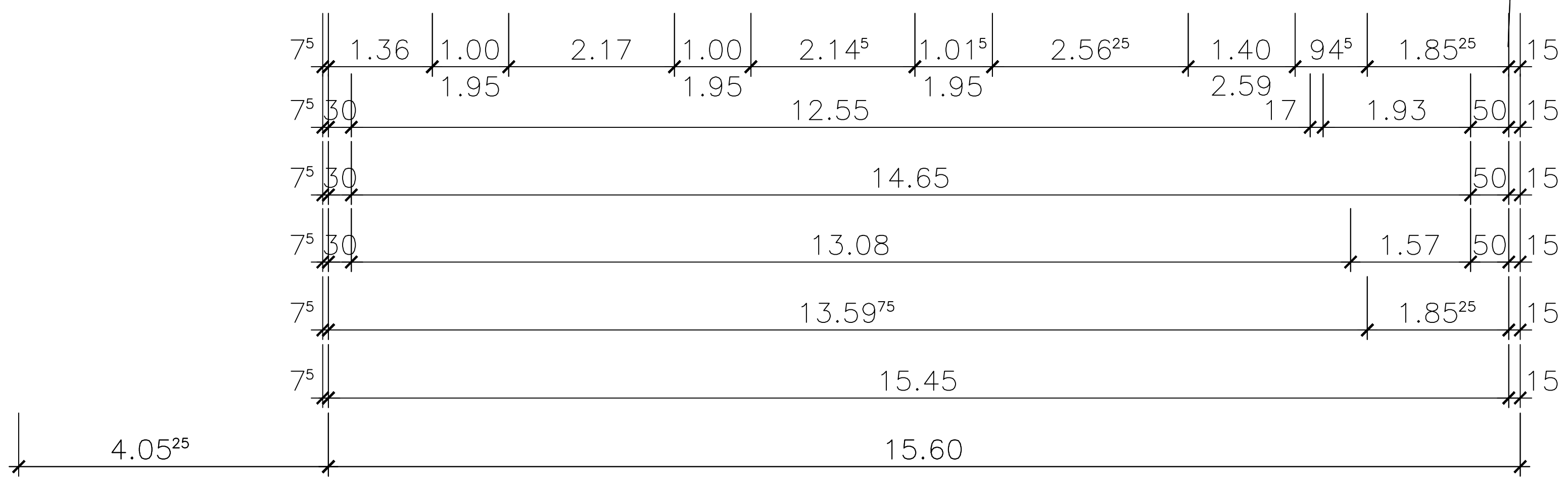
ERDGESCHOSS BESTAND / NEUPLANUNG M 1 : 50
