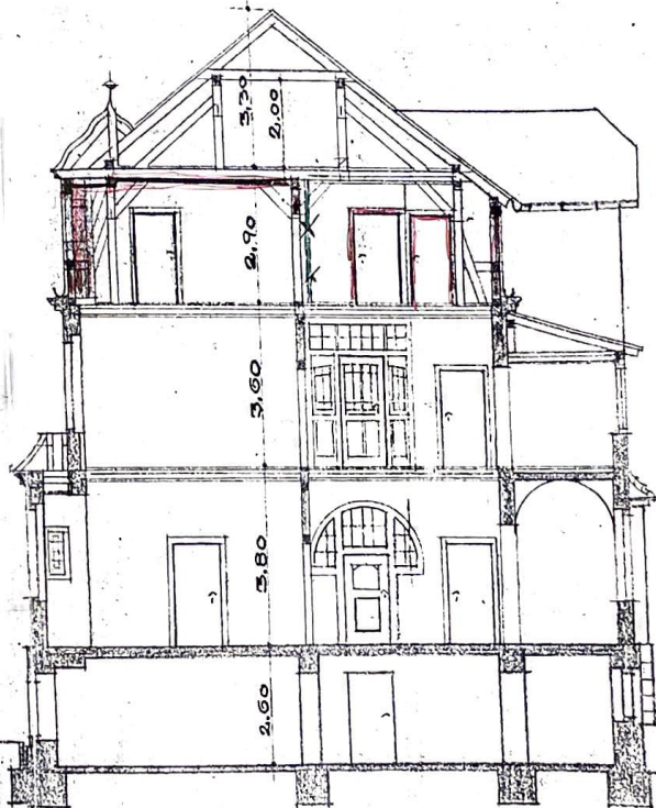
'Schnitt A-B'
