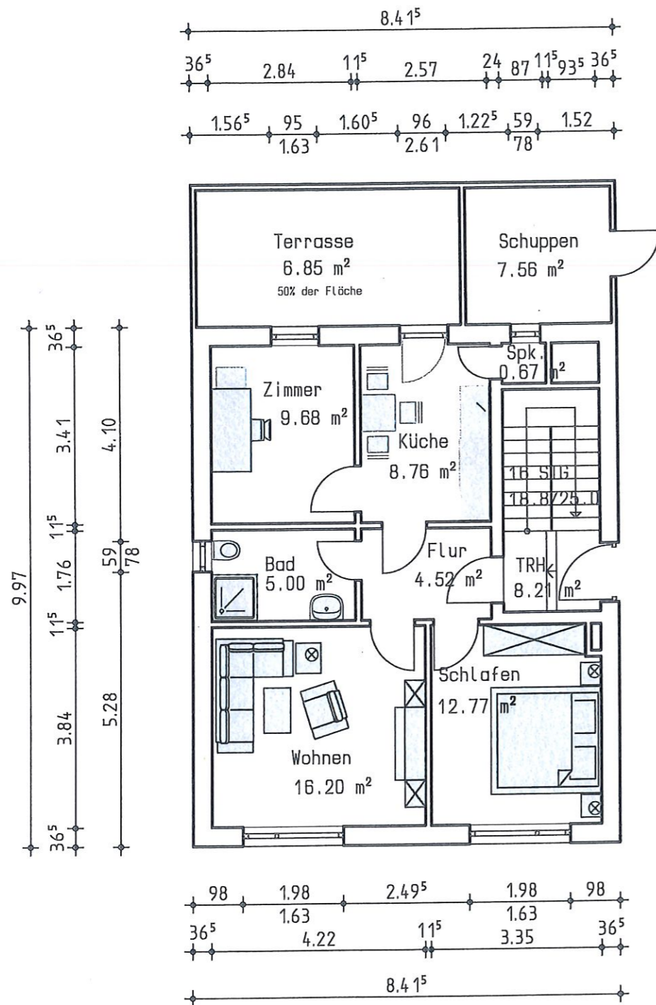
Erdgeschoss
