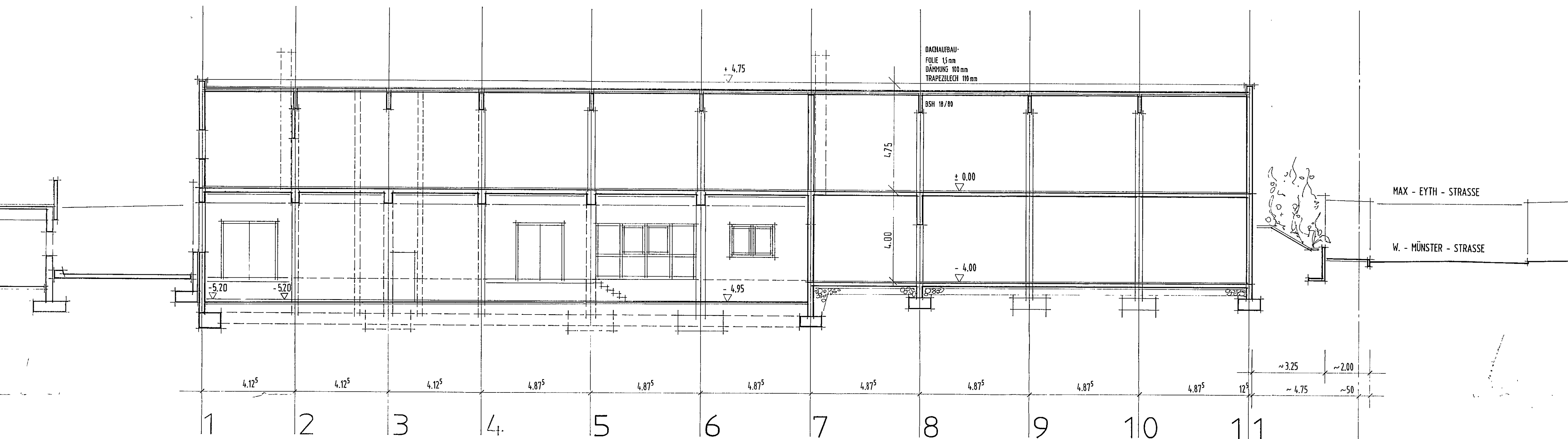
LÄNGSSCHNITT (ACHSE B)
