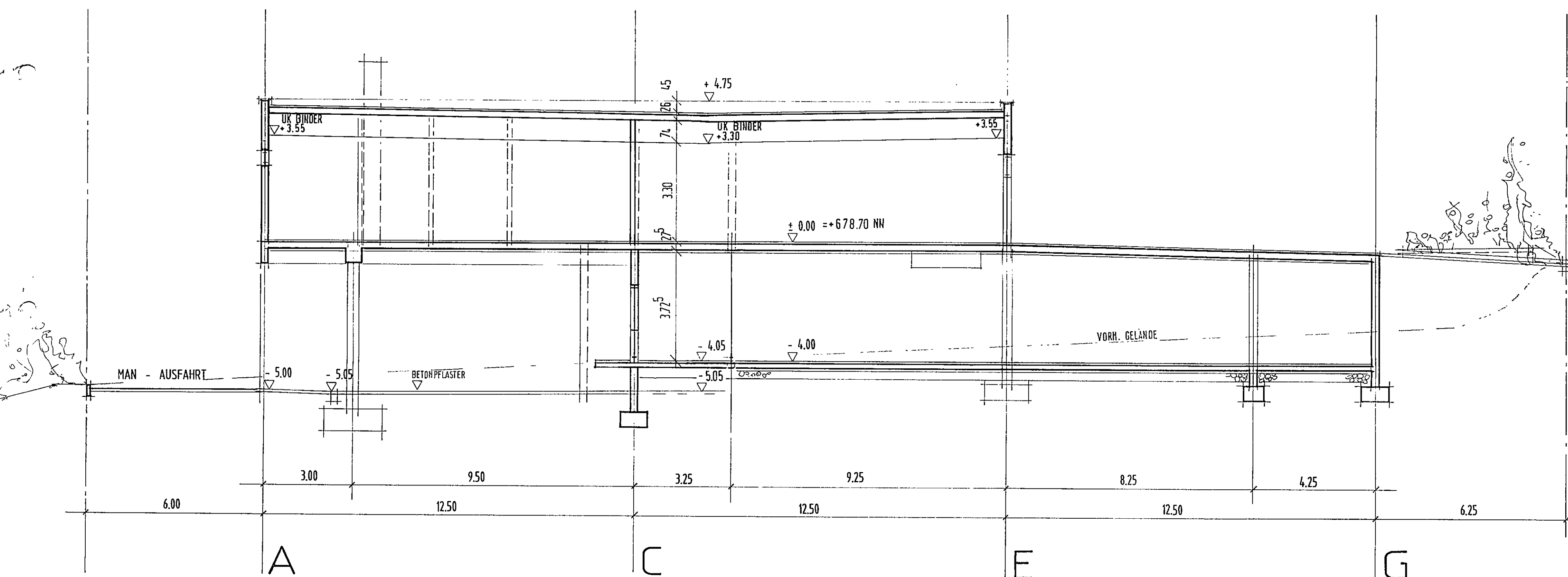
QUERSCHNITT (ACHSE 4/5)
