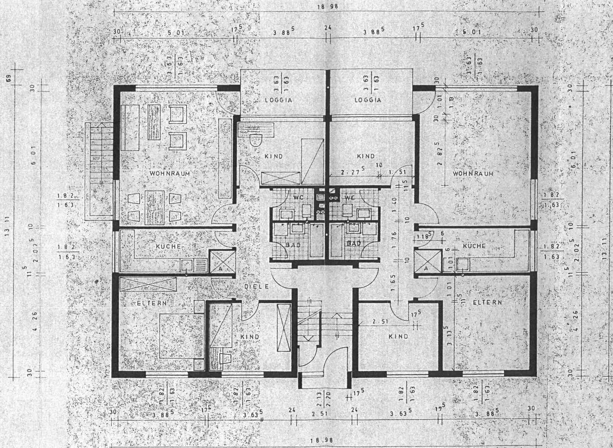
ERDGESCHOSS (OBERGESCHOSS)
