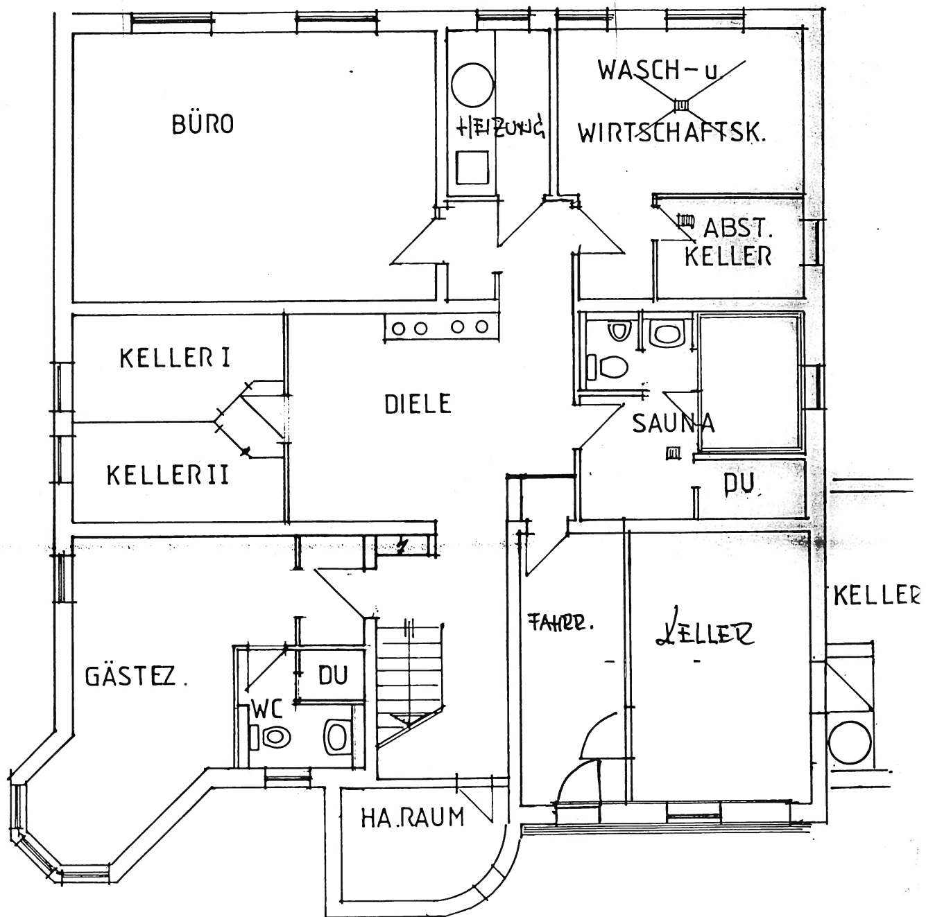
DECKBLATT zum KELLERGESCHOSS
