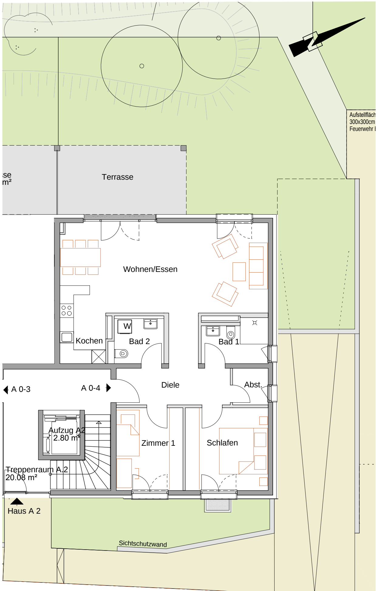
ERDGESCHOSS M. 1:100
