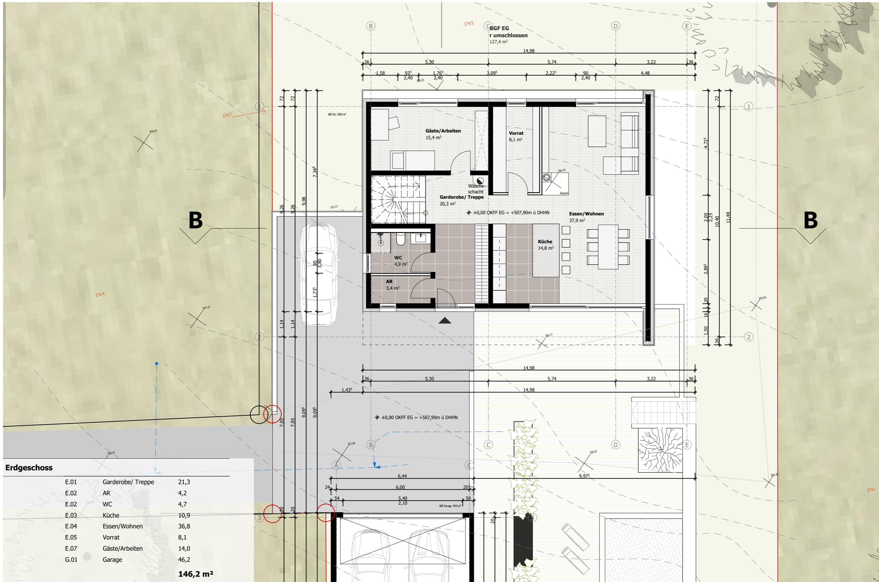
Grundriss Erdgeschoss 1:100
